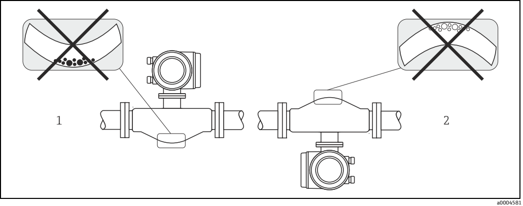
带弯测量管的传感器的安装方向示意图
