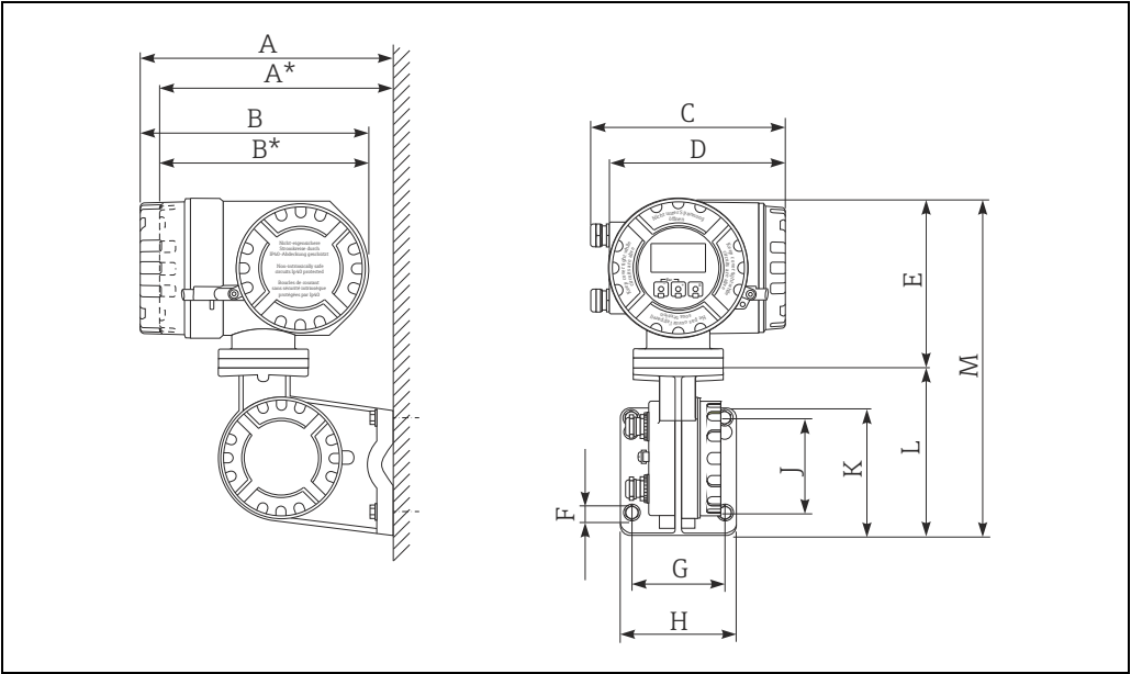
分体式仪表的变送器接线壳 (II2G / 1 区防爆场合 )
