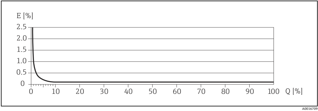
E = 最大测量误差 (% o.r.) ( 图例 : Promass 83S) Q = 流量 (%)
