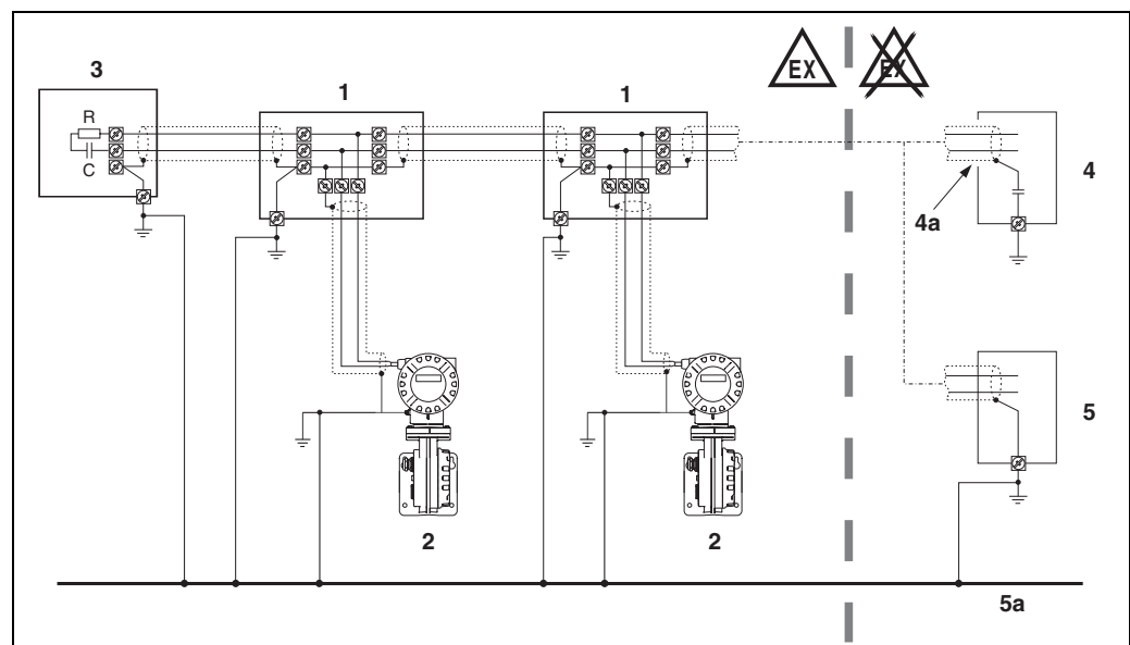
Fig. 3: Exemples pour le raccordement des liaisons équipotentialielles
