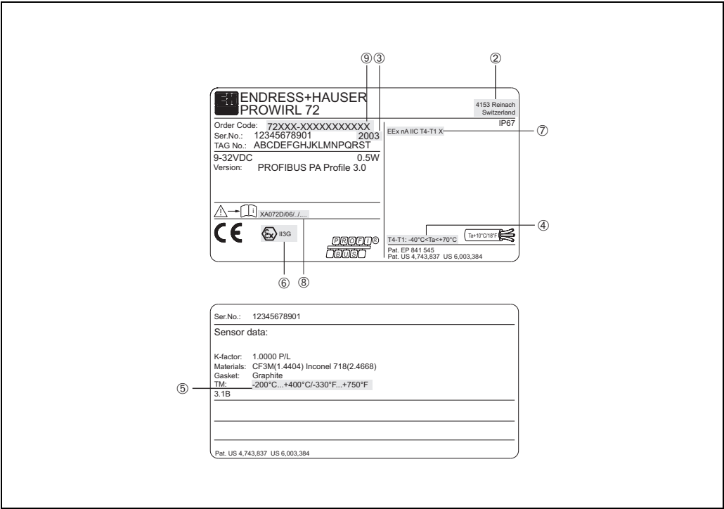
Abb. 4: Typenschild Messumformer und Typenschild Messaufnehmer (Beispiel)
