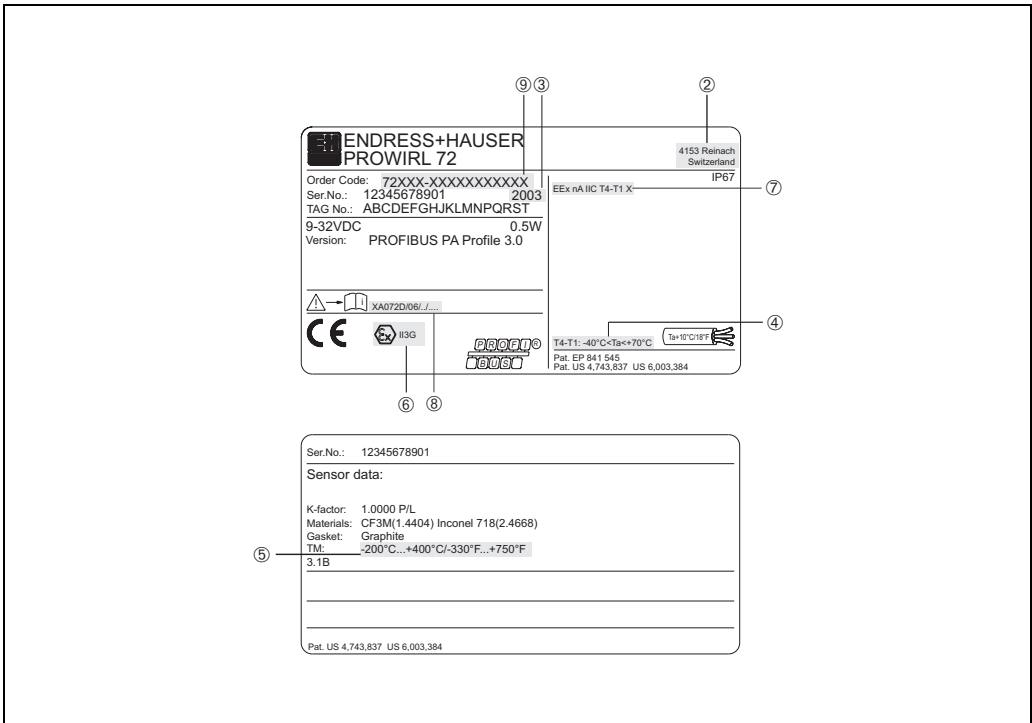
Fig. 4: Plaques signalétiques transmetteur et capteur (exemples))
