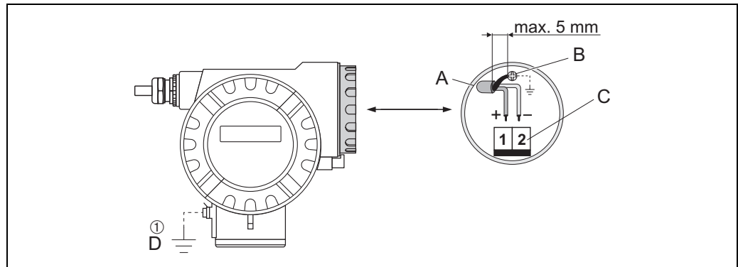
Abb. 1: Elektrischer Anschluss Prowirl 72 PROFIBUS PA bzw. Prowirl 73 PROFIBUS PA
