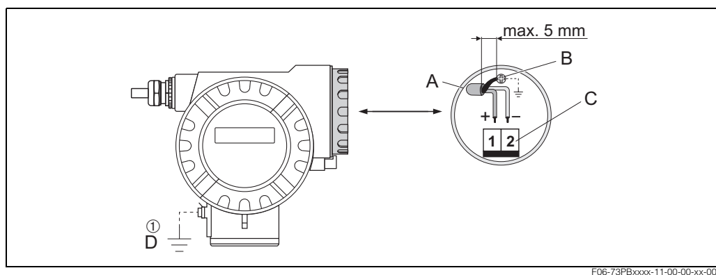
Fig. 1: Raccordements électriques Prowirl 72 PROFIBUS PA resp. Prowirl 73 PROFIBUS PA
