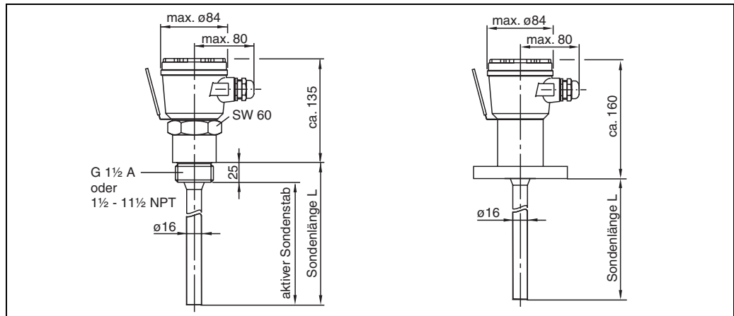
links: Multicap DC 11 mit Einschraubstück rechts: Multicap DC 11 mit Flansch
