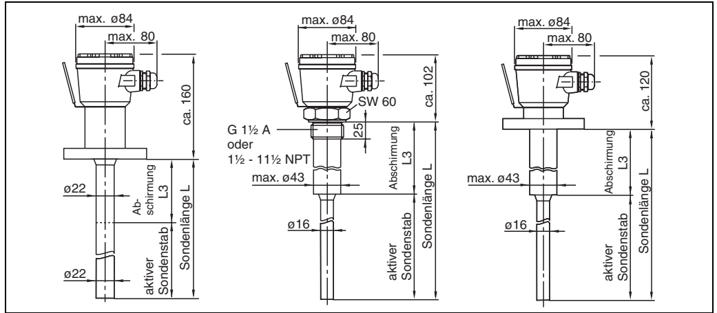
links: Multicap DC 11 mit PTFE-plattiertem Flansch und vollisolierter Abschirmung mitte: Multicap DC 11 mit Einschraubstück und Abschirmung rechts: Multicap DC 11 mit Flansch und Abschirmung
