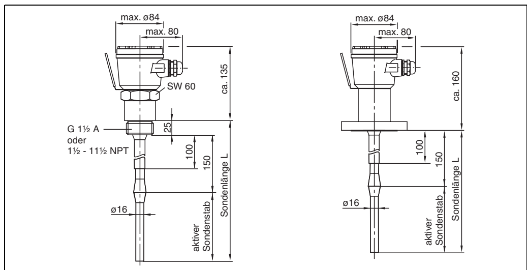
links: Multicap DC 11 mit Einschraubstück und aktiver Ansatzkompensation rechts: Multicap DC 11 mit Flansch und aktiver Ansatzkompensation
