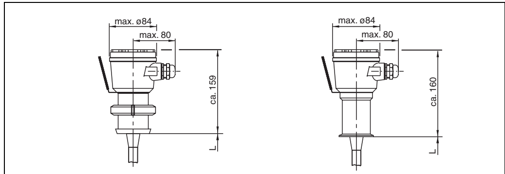
links: Multicap DC 11 mit Milchrohrverschraubung DN 50 rechts: Multicap DC 11 mit Triclamp-Kupplung 2"
