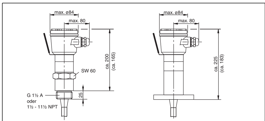
links: Multicap DC 11 mit Einschraubstück und Temperaturreduzierstück rechts: Multicap DC 11 mit Flansch und Temperaturreduzierstück
