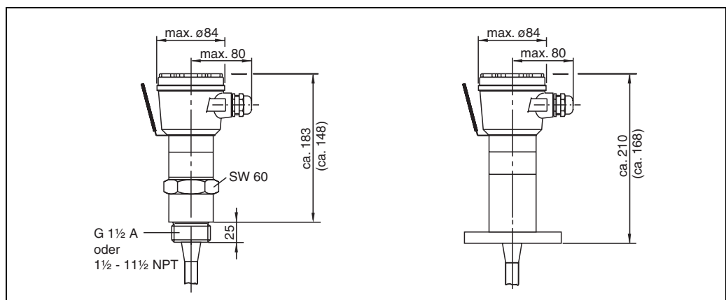
links: Multicap DC 11 mit Einschraubstück und gasdichter Durchführung rechts: Multicap DC 11 mit Flansch und gasdichter Durchführung
