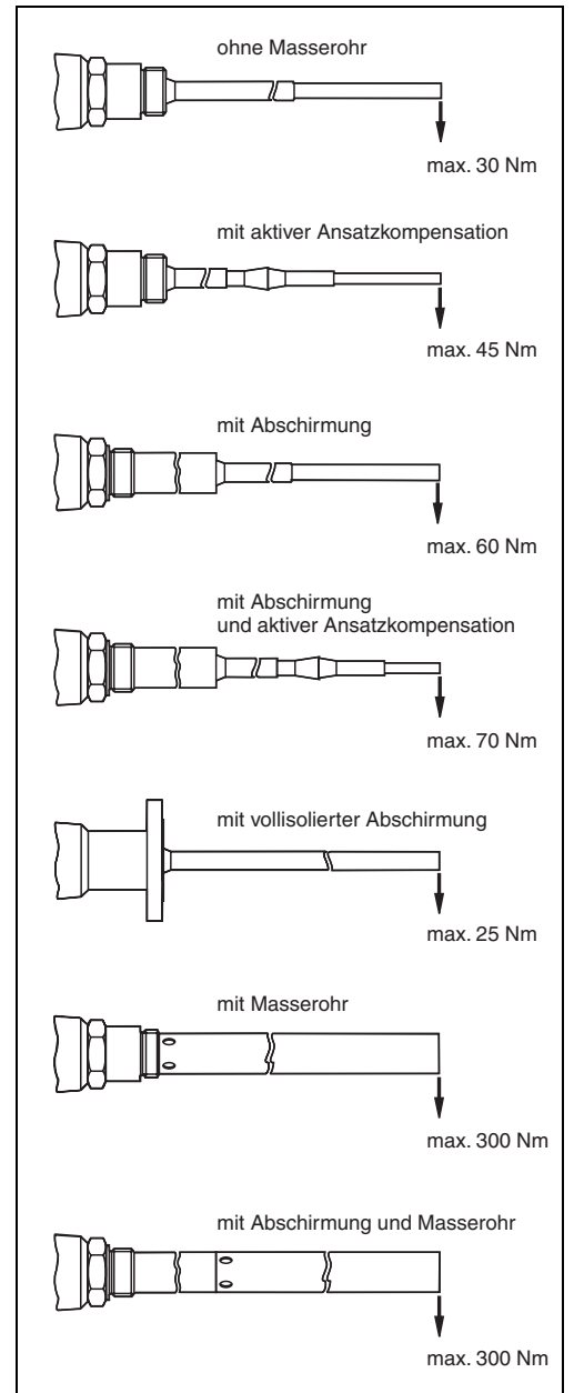
Seitliche Belastbarkeit der Sonde bei 20 °C und statischer Belastung
