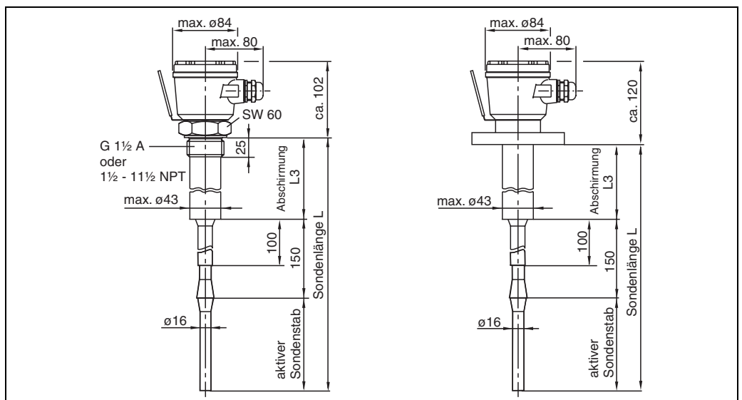
links: Multicap DC 11 mit Einschraubstück, mit Abschirmung und aktiver Ansatzkompensation rechts: Multicap DC 11 mit Flansch, mit Abschirmung und aktiver Ansatzkompensation
