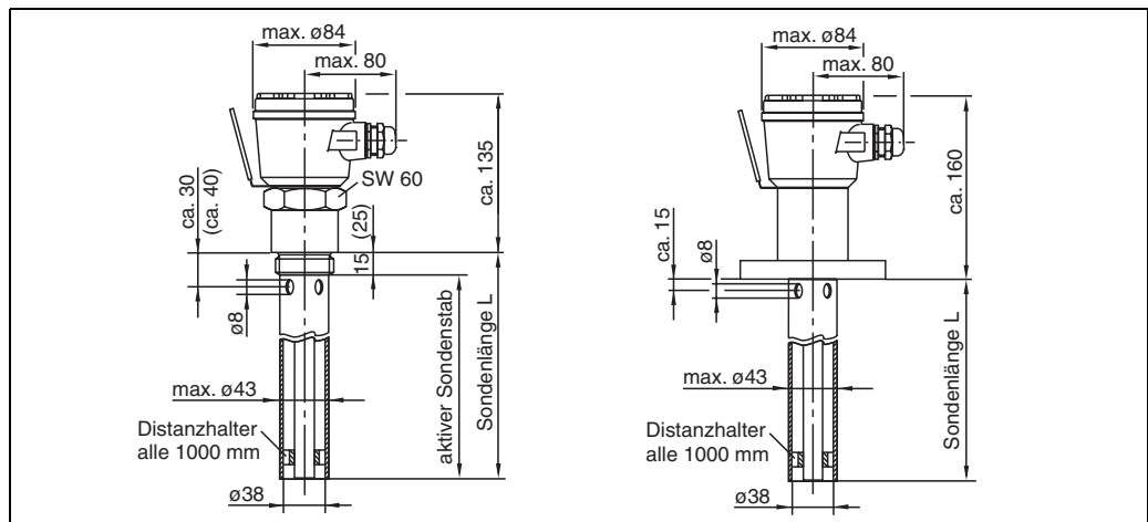
links: Multicap DC 11 mit Einschraubstück G 1 1/2 A und Masserohr (Maße in Klammern gelten für Einschraubstück 1 1/2 - 11 1/2 NPT) rechts: Multicap DC 11 mit Flansch und Masserohr
