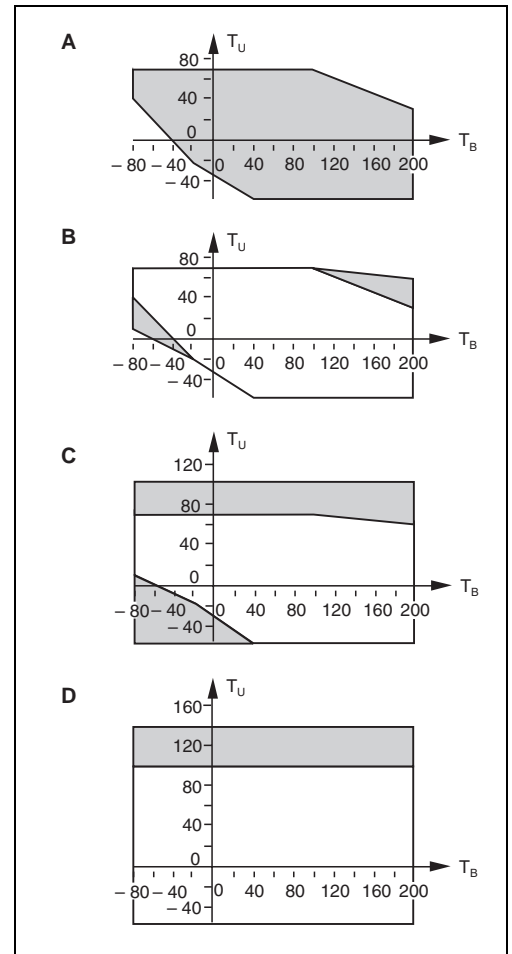
Anwendungsbereiche verschiedener Varianten in Abhängigkeit von Betriebstemperatur und Umgebungstemperatur
