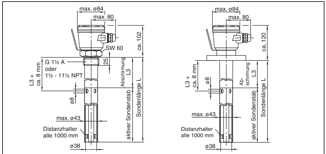
links: Multicap DC 11 mit Einschraubstück, mit Abschirmung und Masserohr rechts: Multicap DC 11 mit Flansch, mit Abschirmung und Masserohr
