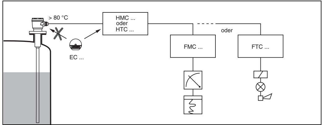
Separate Montage des Elektroneinsatzes bei zu hoher Umgebungstemperatur für das Sondengehäuse
