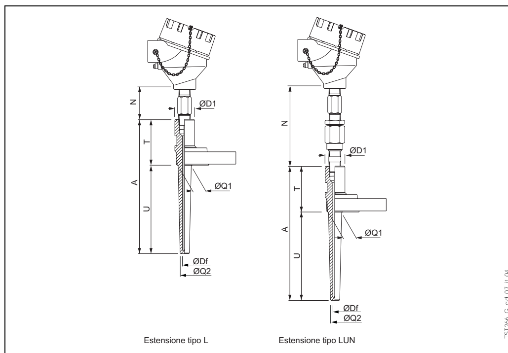
Fig. 1: Indicazioni dimensionali base
