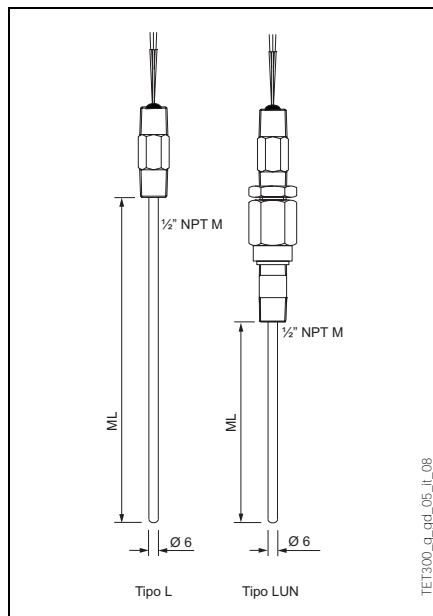
Fig. 8: Sonda di misura
