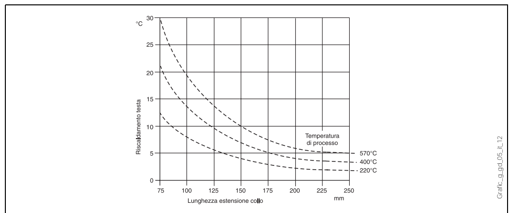
Fig. 6: Riscaldamento della testa conseguente alla temperatura del processo
