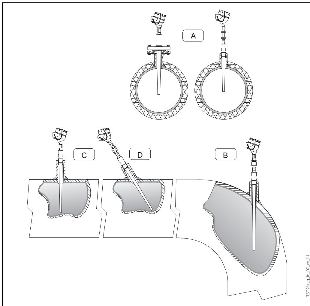
Fig. 3: Installazione in tubature e serbatoi con attacchi al processo flangiate o filettate
