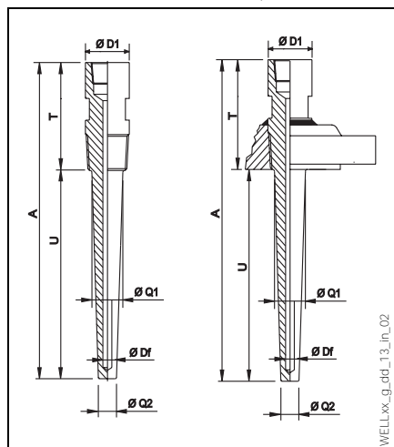
Fig. 7: Pozzetto con attacco al processo filettato o flangiato
