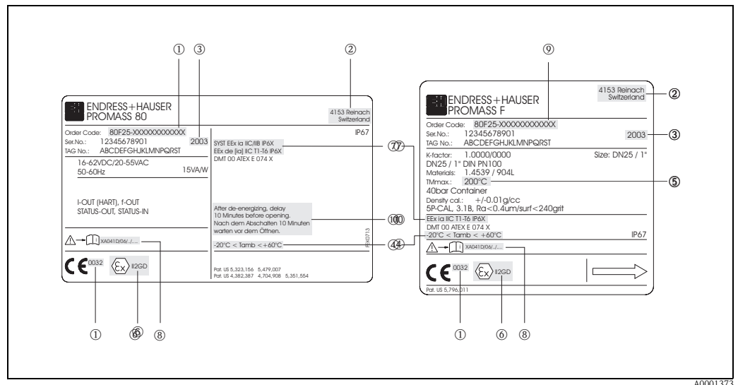
Abb. 5: Typenschild Messumformer und Typenschild Messaufnehmer (Beispiel)
