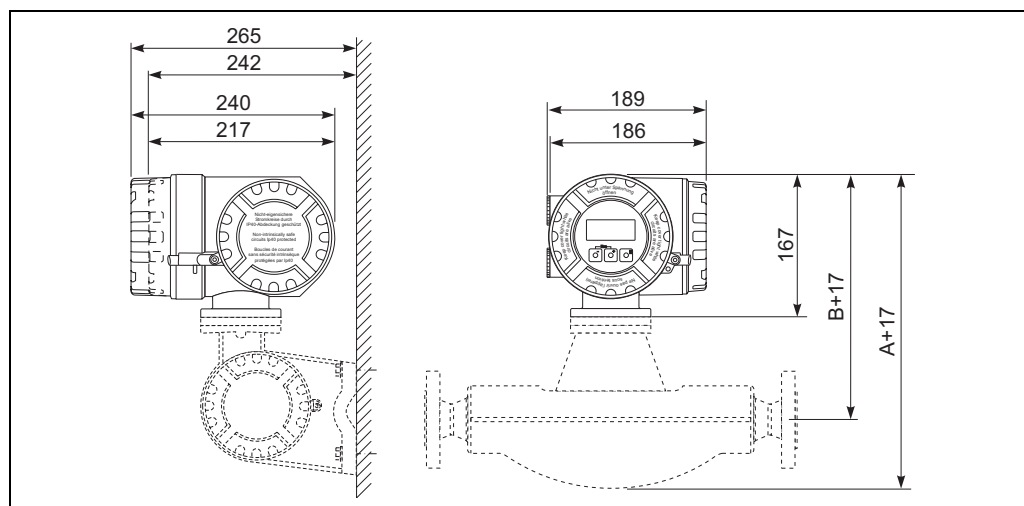
Abb. 4: Abmessungen Ex-Messumformergehäuse
