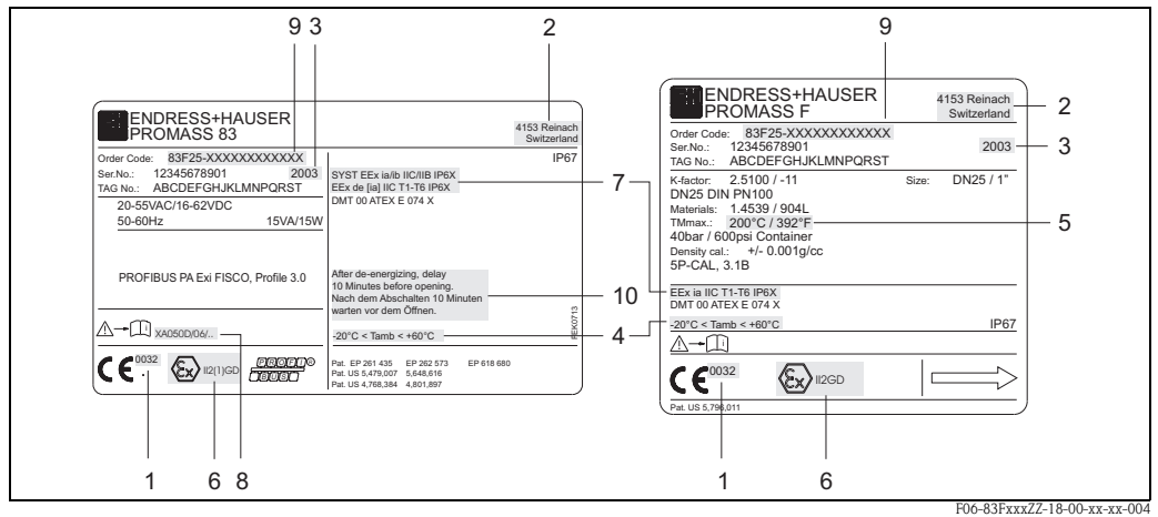
Abb. 5: Typenschild Messumformer und Typenschild Messaufnehmer (Beispiel)
