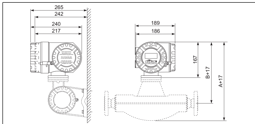
Abb. 4: Abmessungen Ex-Messumformergehäuse
