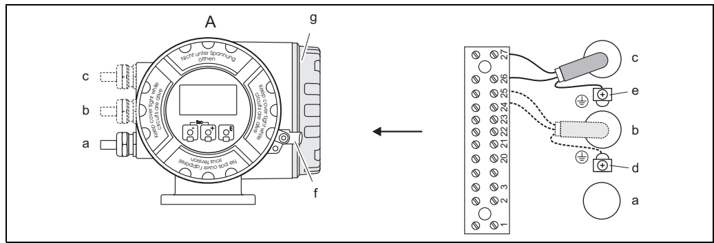
Abb. 2: Anschluss Ein-/Ausgangskreise
