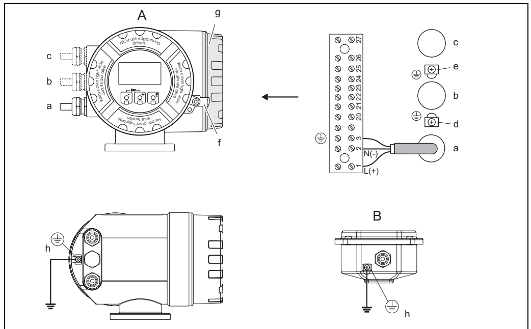
Abb. 1: Anschluss Hilfsenergie und Potentialausgleich A Messumformergehäuse (Kompakt- bzw. Getrenntausführung) B Anschlussgehäuse der Getrenntausführung a Kabel für Hilfsenergie b Spannungsversorgungskabel für externe Terminierung (siehe Abb. 2) c Buskabel PROFIBUS DP/PA (siehe Abb. 2) d Erdungsklemme für Schutzleiter e Erdungsklemme für das Spannungsversorgungskabel für externe Terminierung und der PROFIBUS DP/PA Leitung f Sicherungskralle g Anschlussklemmenraumdeckel h Schraubklemme zum Anschluss an den Potentialausgleich
