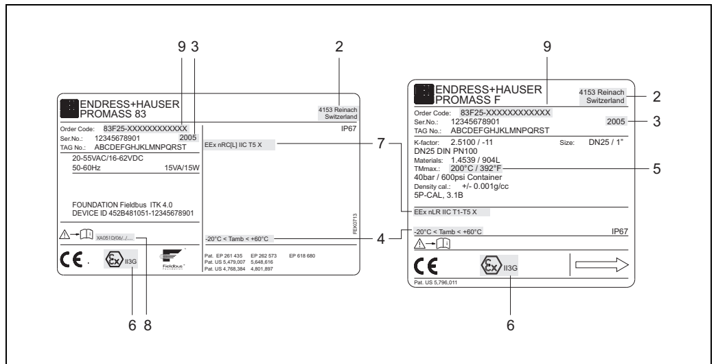
Abb. 4: Typenschild Messumformer und Typenschild Messaufnehmer (Beispiel)
