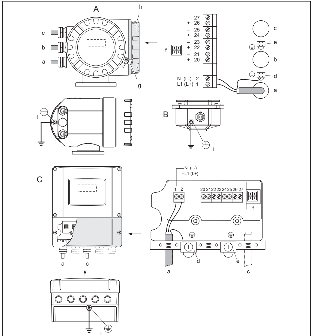
Abb. 1: Anschluss Hilfsenergie
