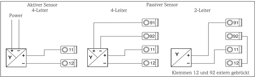
Abb. 8: Anschluss Sensor, Messumformerspeisung und Universaleingang
