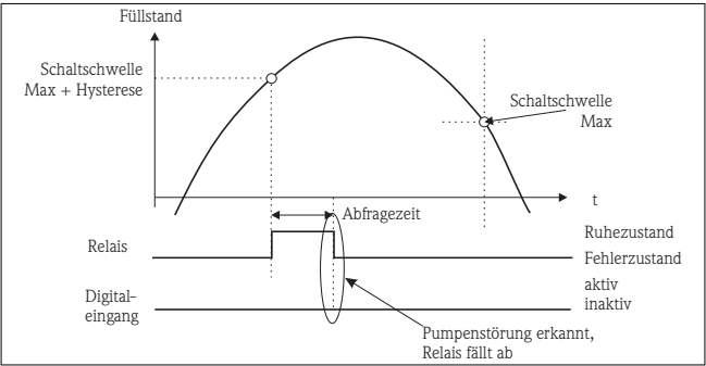
Abb. 15: Pumpenüberwachung, Pumpenstörung
