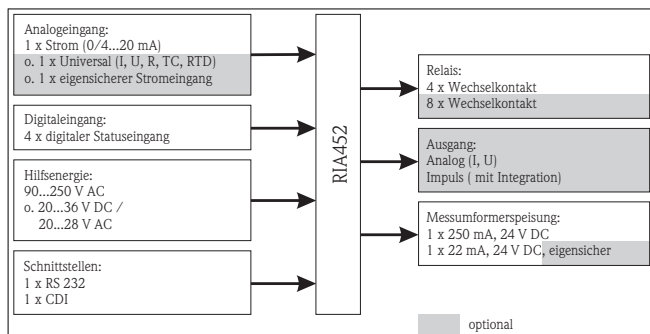
Abb. 1: Blockschaftbild RIA452
