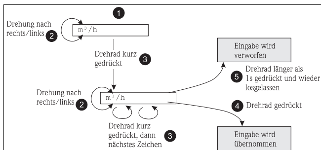
Abb. 13: Texteingabe RIA452
