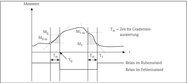
Abb. 18: Betriebsart Grad
