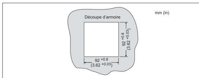
Fig. 3 : Découpe d'armoire électrique (indications en mm)
