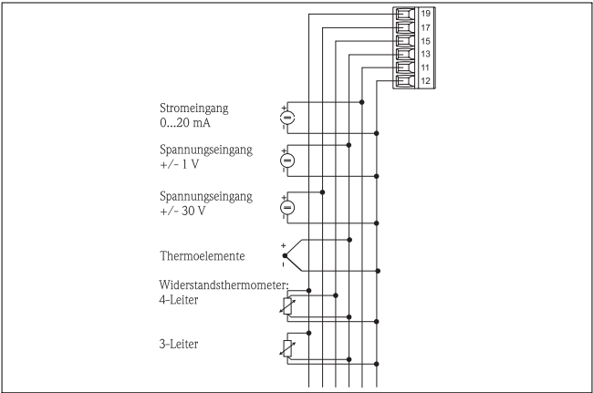
Abb. 5: Klemmenbelegung Universaleingang
