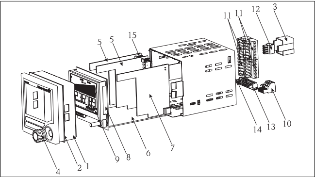
Abb. 21: Ersatzteile RIA452
