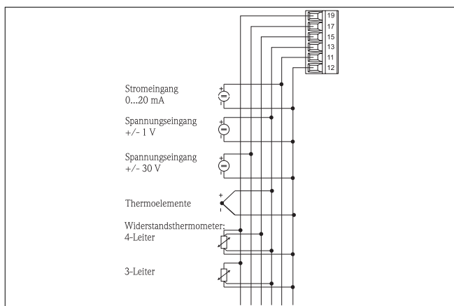
Abb. 23: Klemmenbelegung Universaleingang
