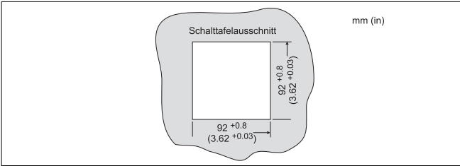
Abb. 25: Schalttafelausschnitt
