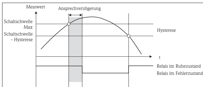
Abb. 19: Ansprechverzögerung
