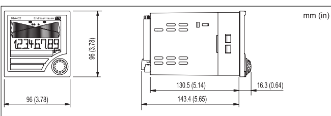
Fig. 24 : Indications en mm
