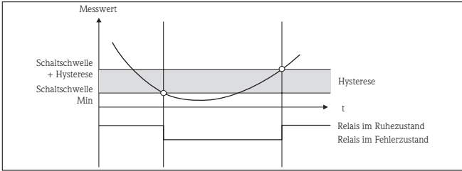
Abb. 16: Betriebsart Min
