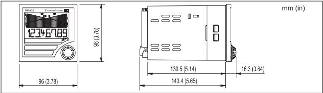
Abb. 24: Abmessungen des RIA452
