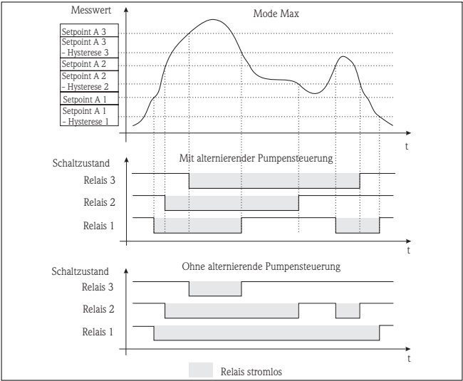
Abb. 20: Alternierende Pumpensteuerung
