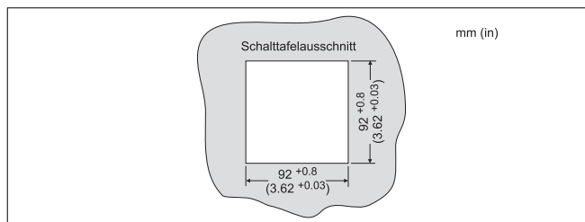
Abb. 3: Schalttafel Ausschnitt (Angaben in mm)
