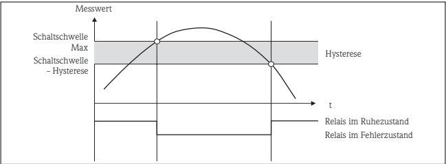
Abb. 17: Betriebsart Max
