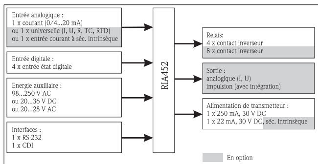
Fig. 1 : Schéma électrique RIA452
