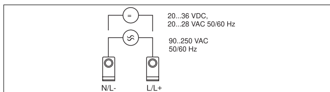
Abb. 6: Anschluss Hilfsenergie
