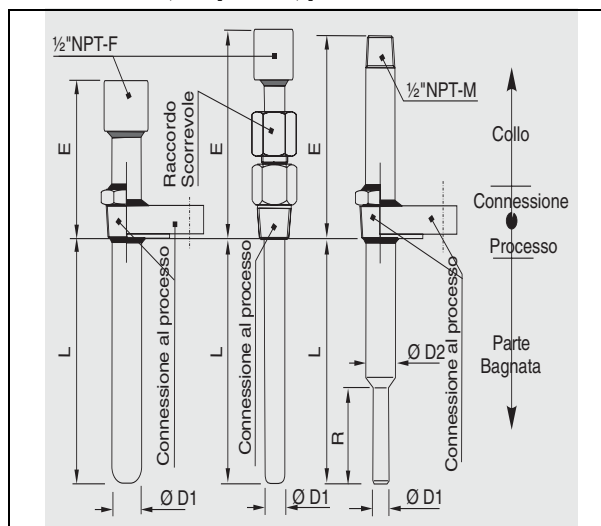
Fig. 6: Pozzetto con connessione al processo filettata o flangiata
