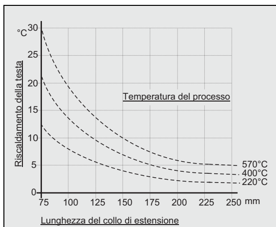
Fig. 5:Riscaldamento della testa conseguente alla temperatura del processo
