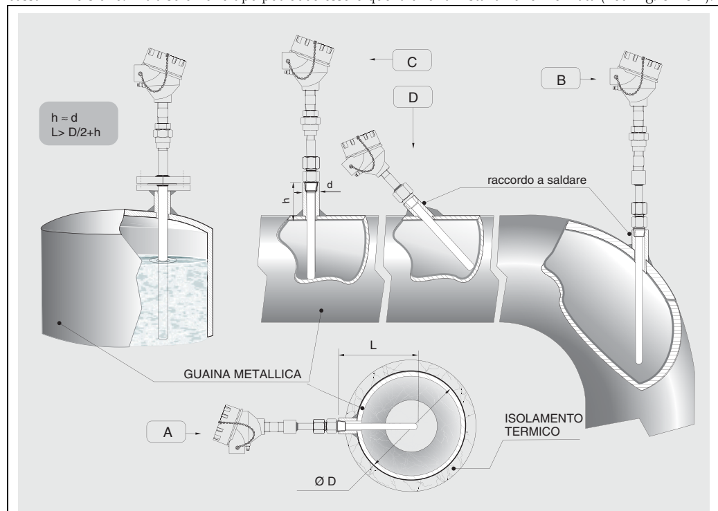
Fig. 3: Esempi di installazione
