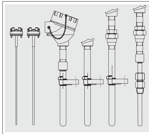
Fig. 1: TR 66 con i vari tipi di connessioni al processo e le parti terminali della sonda
