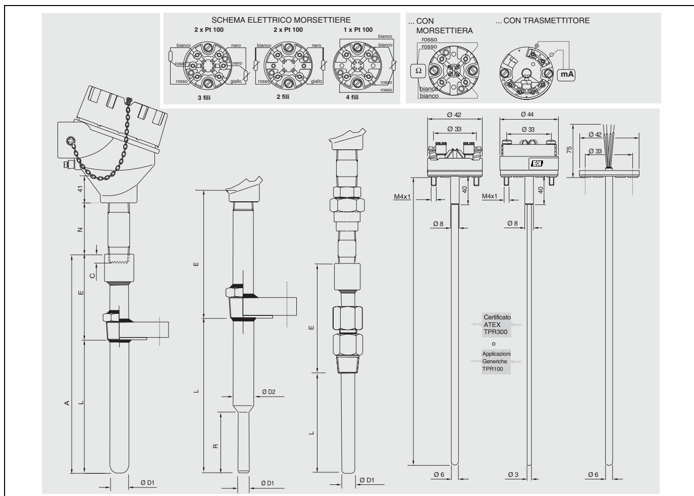
Fig. 7: Componenti funzionali, schemi elettrici standard (morsettiere in ceramica)
