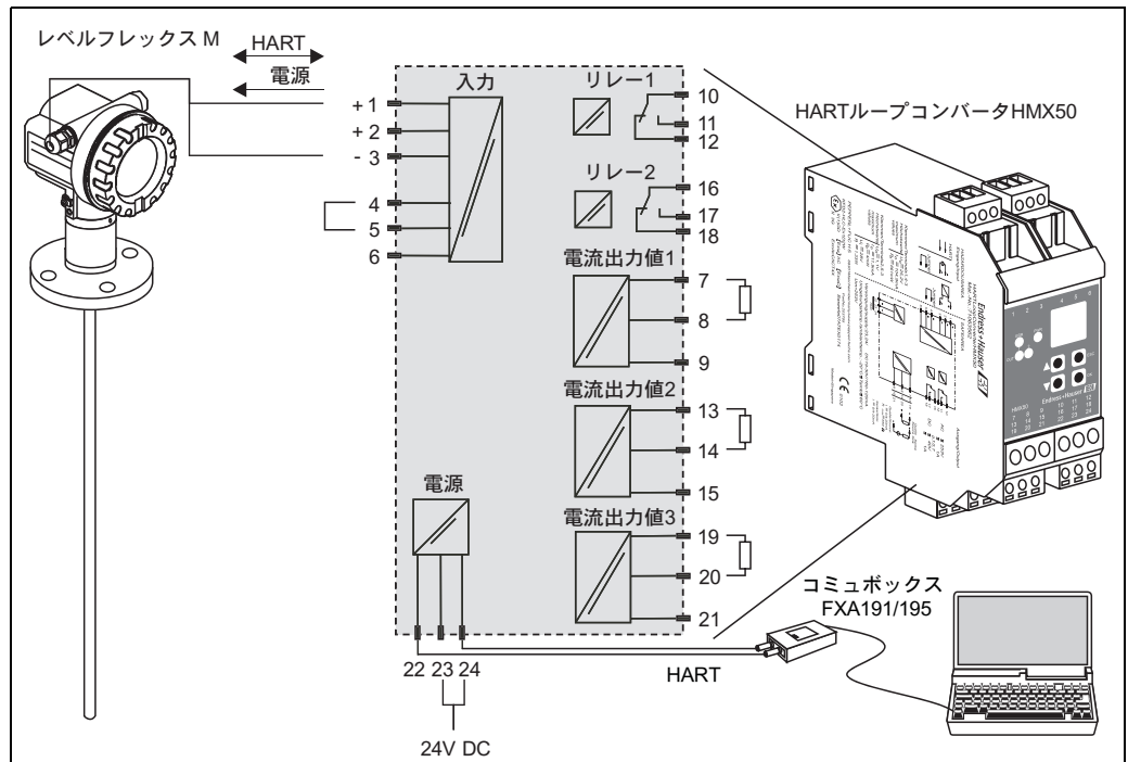
図 2 HART ループコンバータ HMX50 の接続図 (例: 受動 2 線装置と電流出力 (電源として接続))
