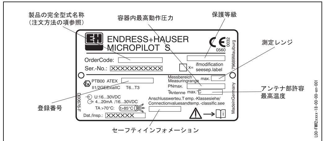
図1 マイクロパイロット S FMR 533、銘板上の記載事項
