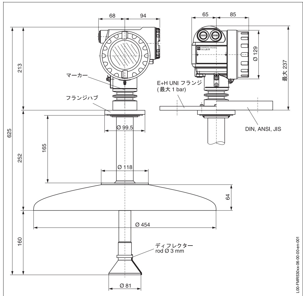
図4 マイクロパイロット S FMR 533 の寸法
