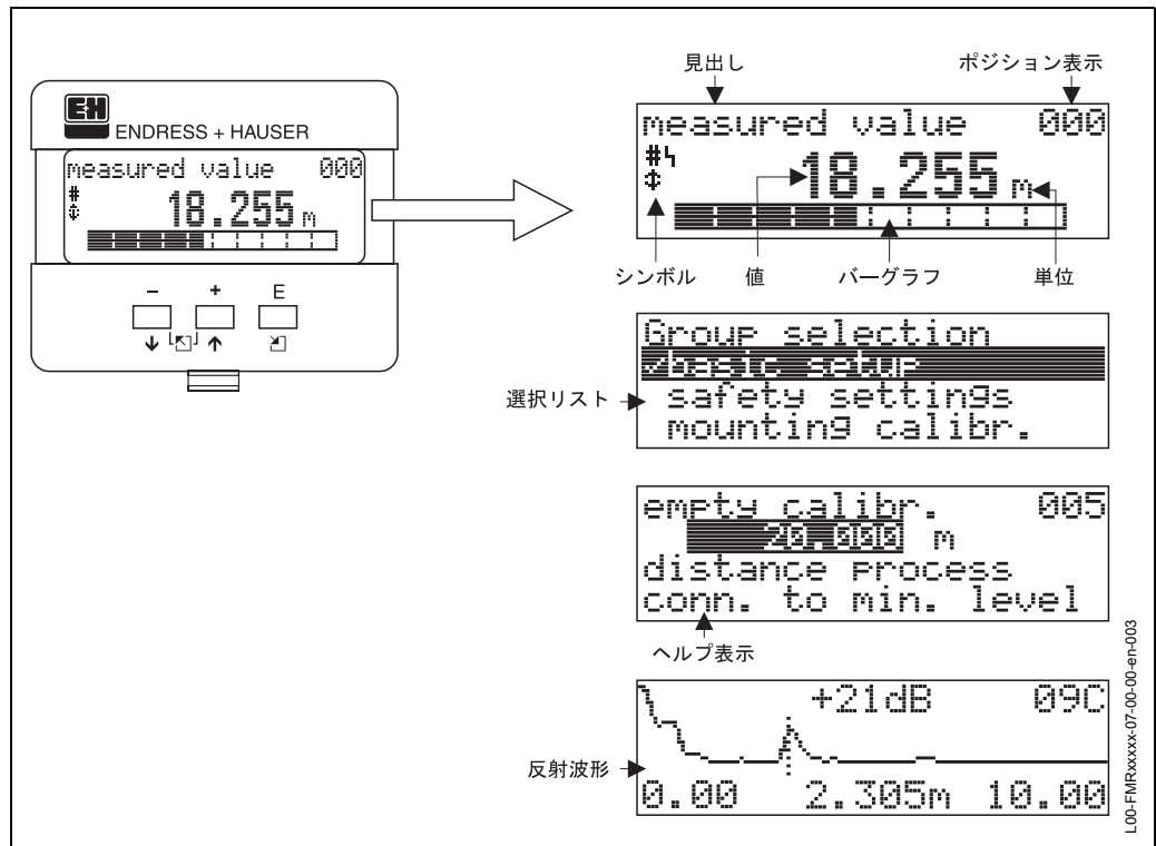
図4 表示ディスプレイ
