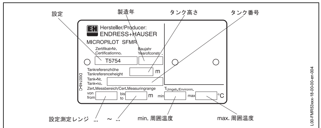
図2 マイクロパイロット S FMR 533、保税アプリケーション用 NMi タイプのプレート上の記載事項 (例)
