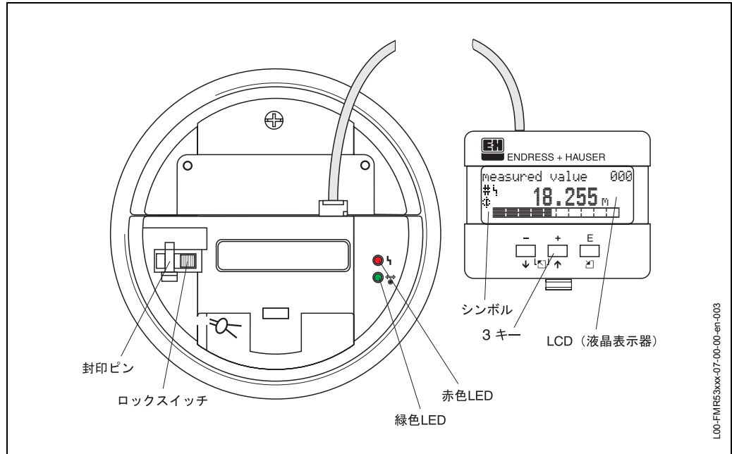
図3 表示ディスプレイと操作エレメントのレイアウト
