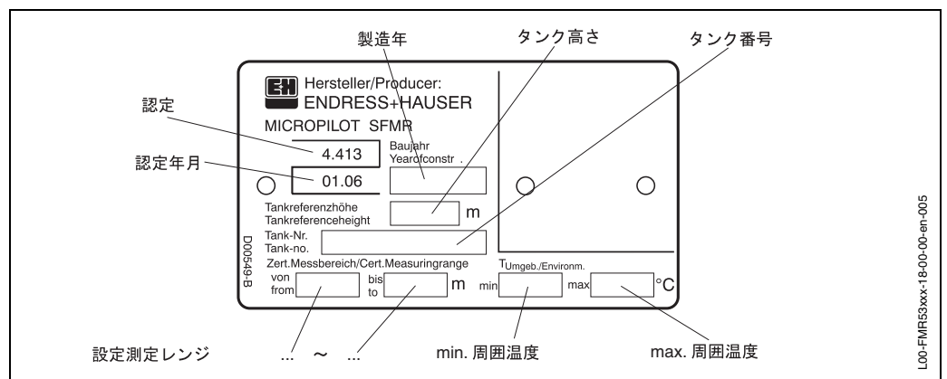
図3 マイクロパイロット S FMR 533、保税アプリケーション用 PTB タイプのプレート上の記載事項 (例)
