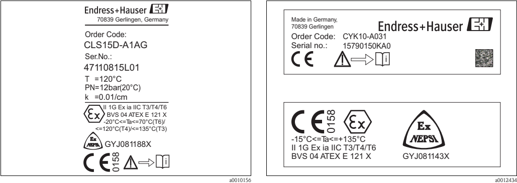
Abb. 2: Typenaufdruck Sensoren CLSxxD (Beispiel) / Type stamp of CLSxxD sensors (example) / Marquage du type de cellules CLSxxD (exemple) Abb. 3: Kabelkennzeichnung / Cable designation / Marquage du câble
