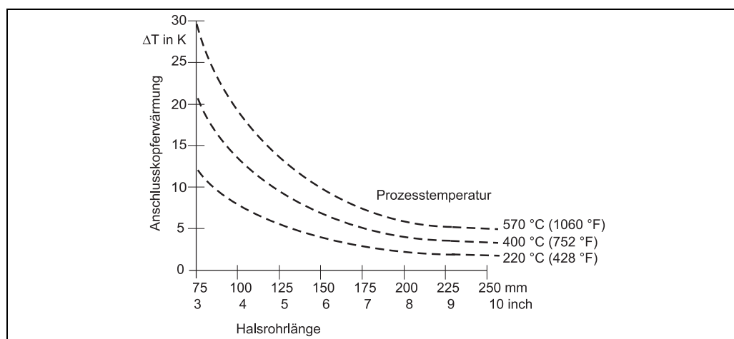
Erwärmung des Anschlusskopfes in Abhängigkeit von der Prozesstemperatur. Temperatur im Anschlusskopf = Umgebungstemperatur 20 °C (68 °F) + ΔT
