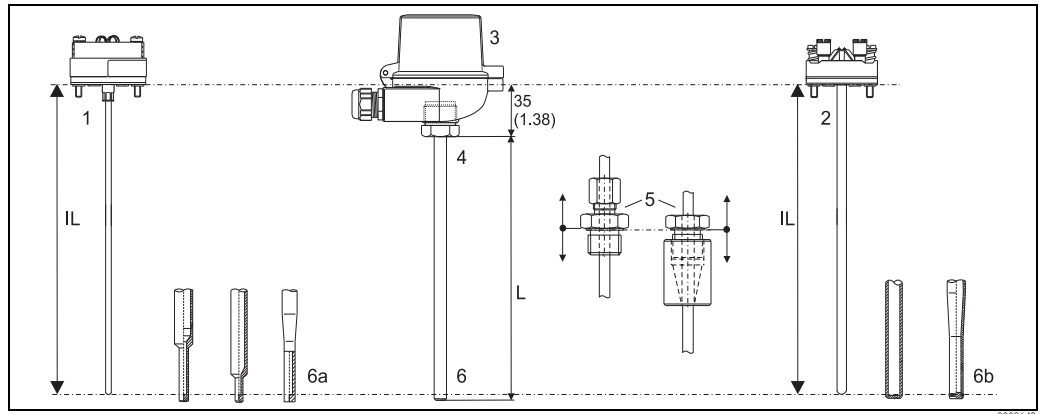
Bauform des Omnigrad M TR12
