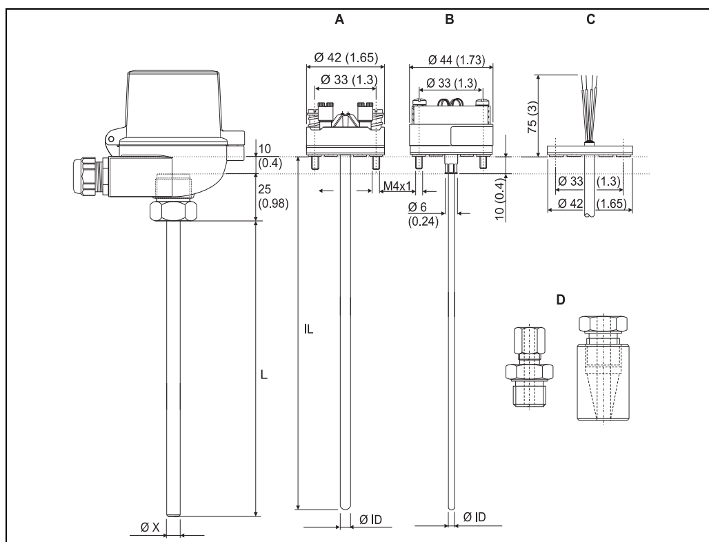
Abmessungen Omnigrad M TR12
