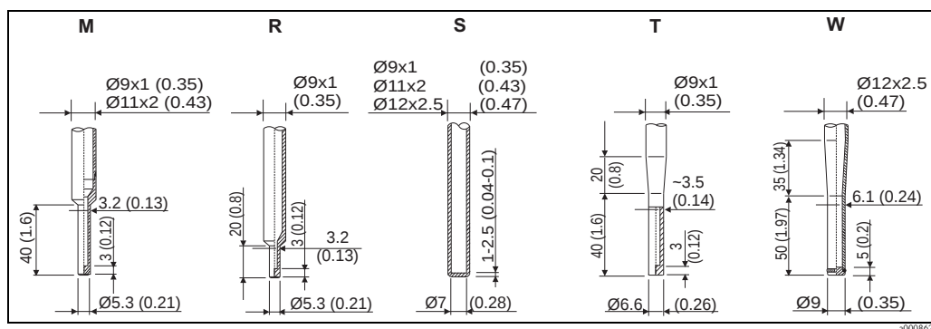
Verfügbare Schutzrohrspitzen (reduziert, gerade oder verjüngt). Maximale Oberflächenrauigkeit Ra \leq 0,8 \mu\text{m} (31.5 \mu\text{in} )
