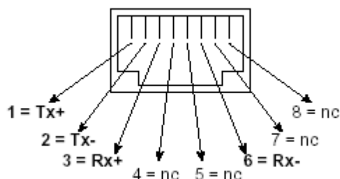
Fig. 8: Connettore a spina RJ45 (assegnazione AT&T256)
