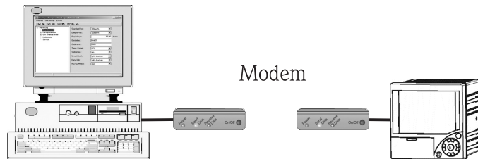
Fig. 14: Connessione del modem al registratore e al PC
