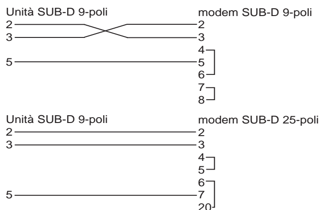
Fig. 13: Assegnazione del cavo modem
