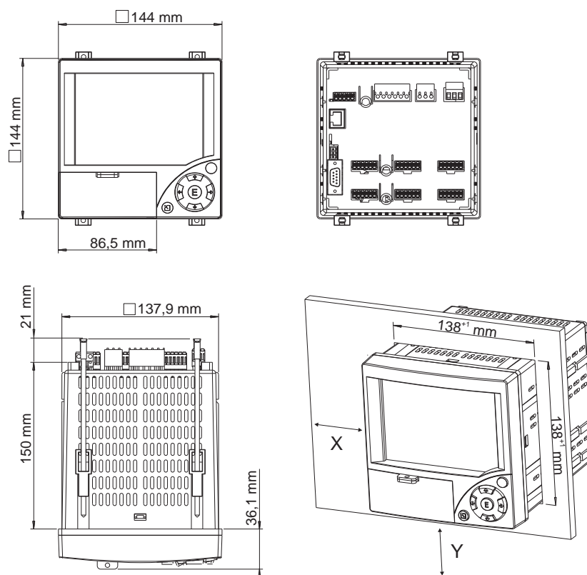
Fig. 3: Installazione a fronte quadro e dimensioni di montaggio
