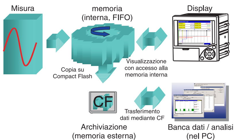
Fig. 55: Rappresentazione schematica della registrazione delle misure
