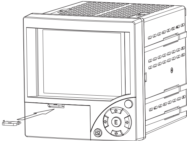
Fig. 4: Inserimento della piastra di blocco
