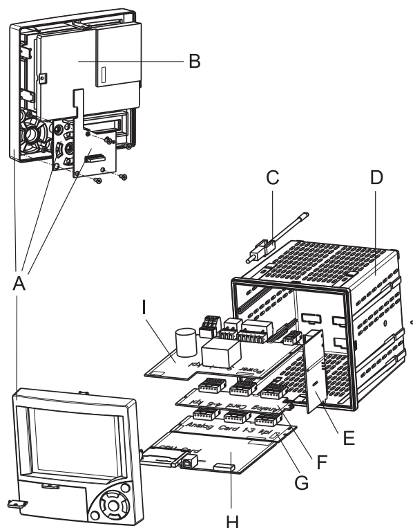
Fig. 61: Schema delle parti di ricambio
