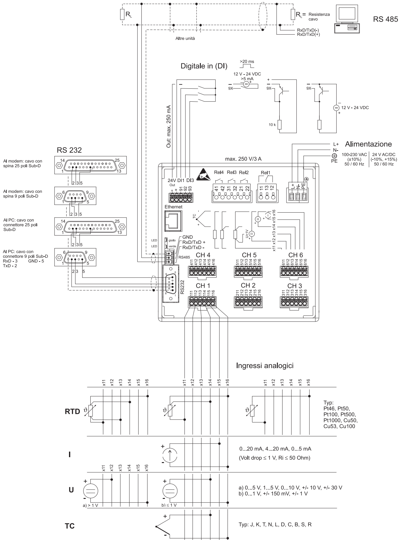
Fig. 5: Schema di cablaggio
