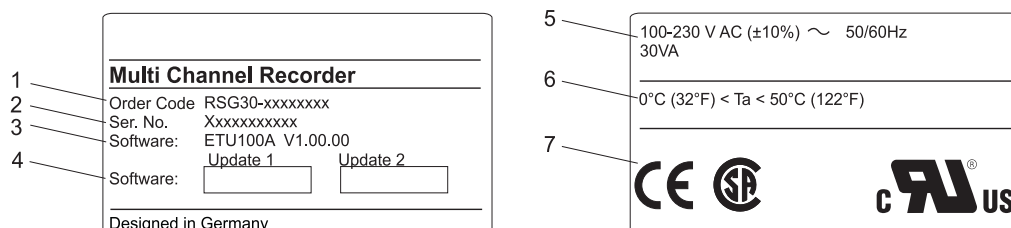
Fig. 2: 1. Codice di ordinazione 2. Numero seriale 3. Versione software 4. Campi didascalici per gli aggiornamenti software installati 5. Tensione, frequenza di rete, rilevazione prestazioni 6. Campo temperatura ambiente 7. Accettazione/inmatricolazione apparecchi
