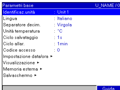
Fig. 21: Configurazione parametri di base
