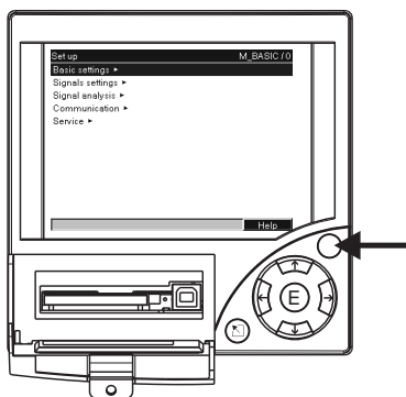
Fig. 10: Variante tasto "Softkey" (ad es. per richiamare la funzione interna di Aiuto in modalità setup)
