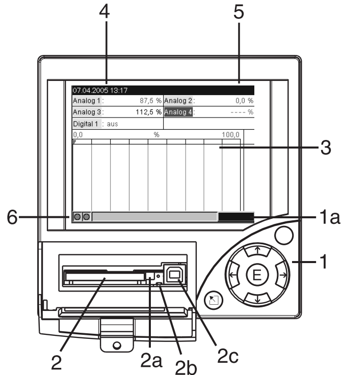
Fig. 11: Display/elementi operativi del registratore
