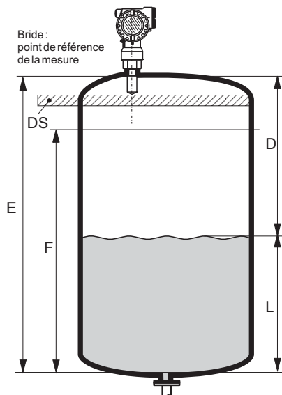
Mesure de niveau dans les liquides
