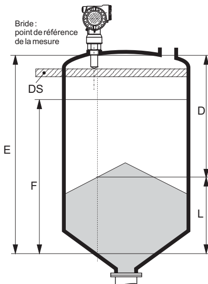
Mesure de niveau dans les solides
