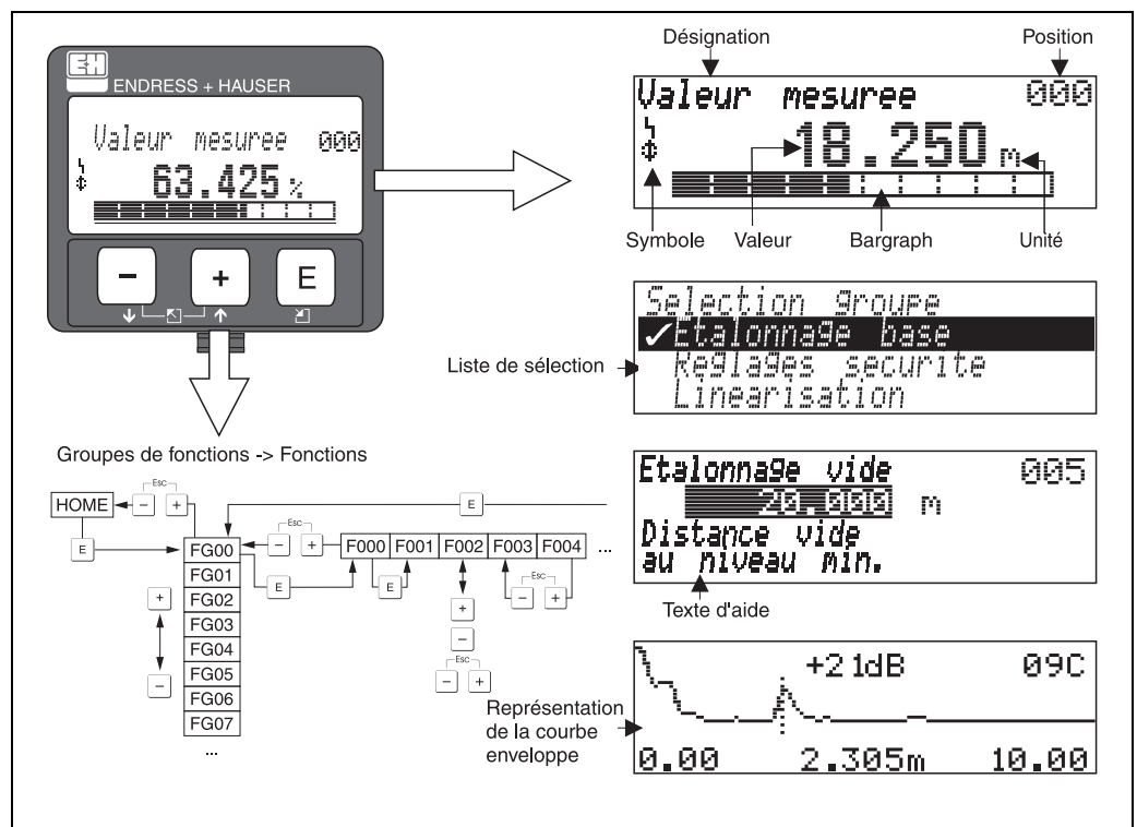
Fig. 2 : Afficheur
