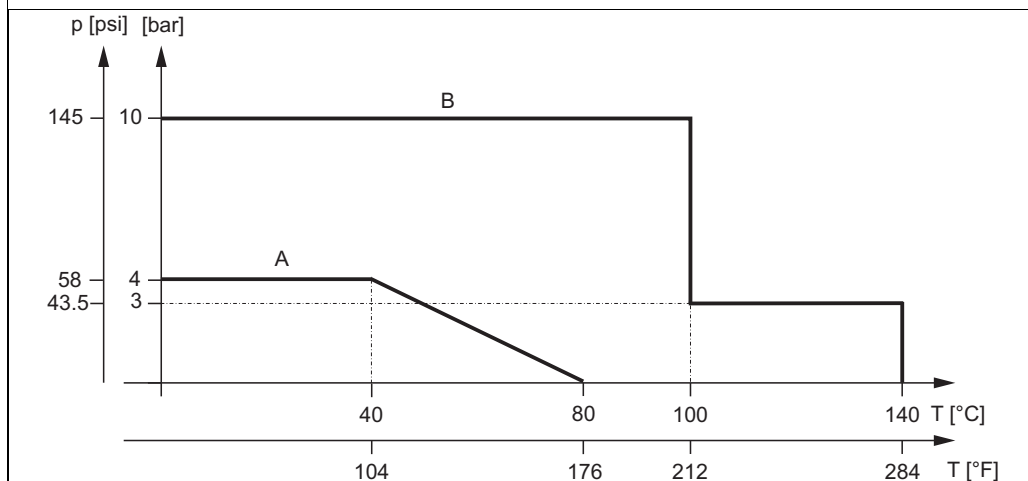
Fig. 26: Pressure-temperature diagramm
