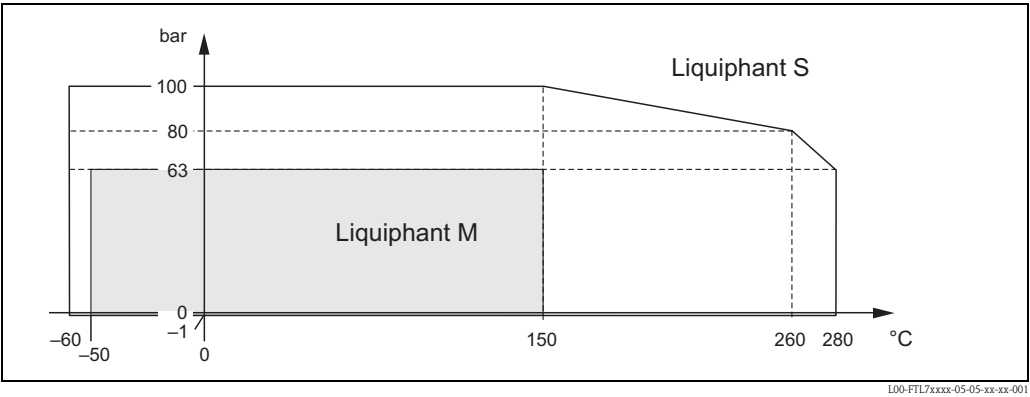
高压滑动套管的压力 - 温度曲线
