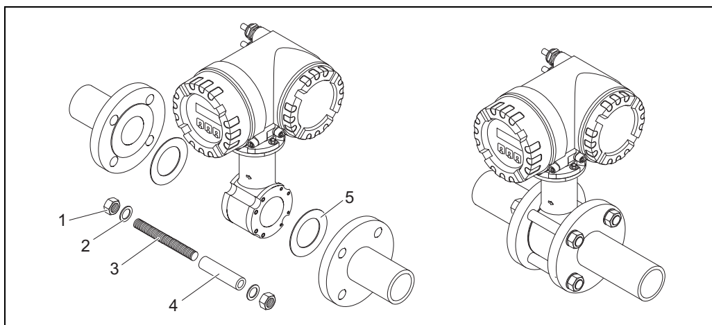
传感器的安装示意图
