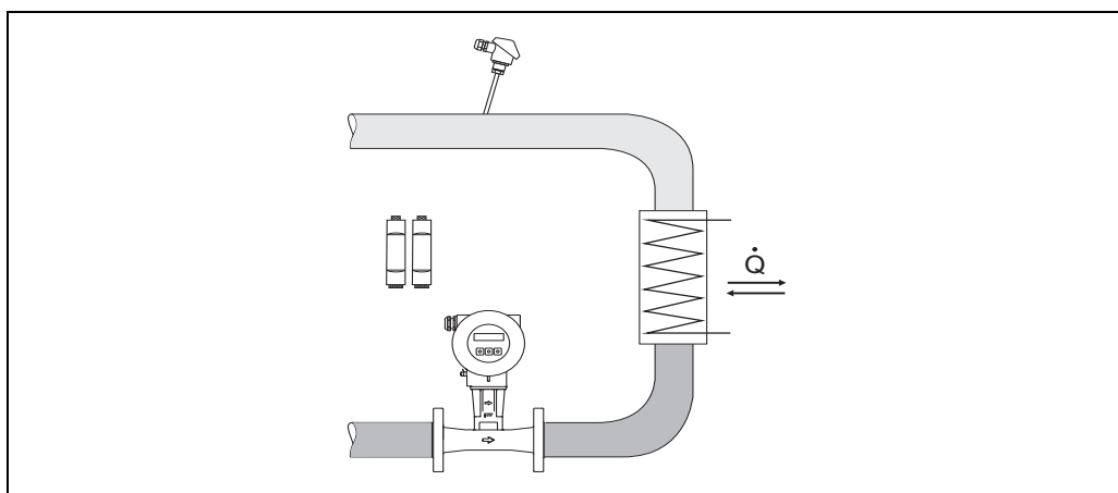
饱和蒸汽和水的换热测量系统布局示意图
