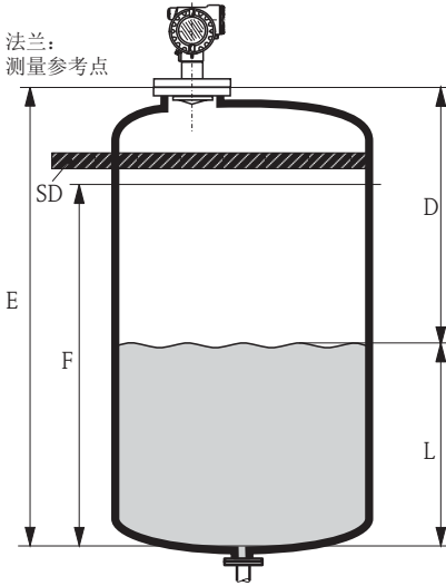
液位测量
