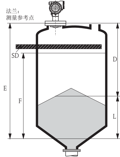
料位测量
