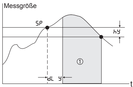
Wirkungsweise der Ansprechverzögerung dL \Delta dL \Delta
