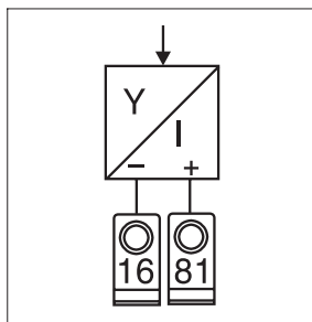
Entrée courant avec alimentation pour transmetteur
