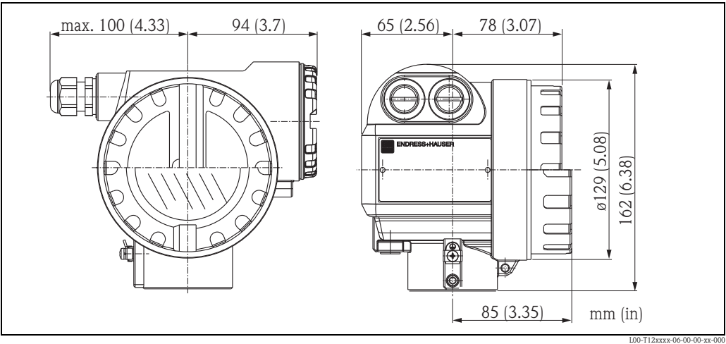
T12 外壳 (铝)
