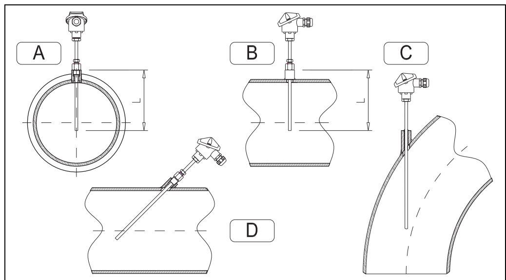
图 4: 安装示意图
