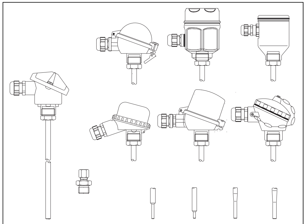
图 1: TC12 示意图，多种表头、过程连接和热保护套管末端部件
