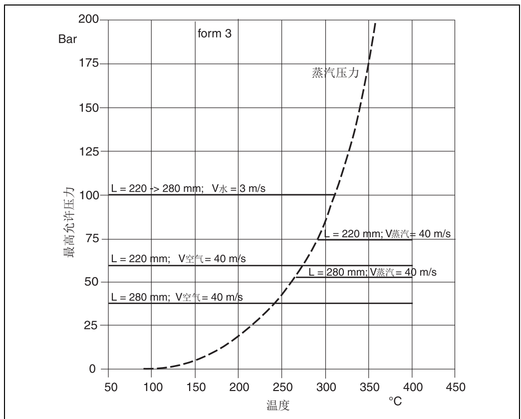
图 3: 压力 - 温度曲线, 适用于 \varnothing 12 mm 锥管型热保护套管, 不锈钢 316Ti/1.4571
