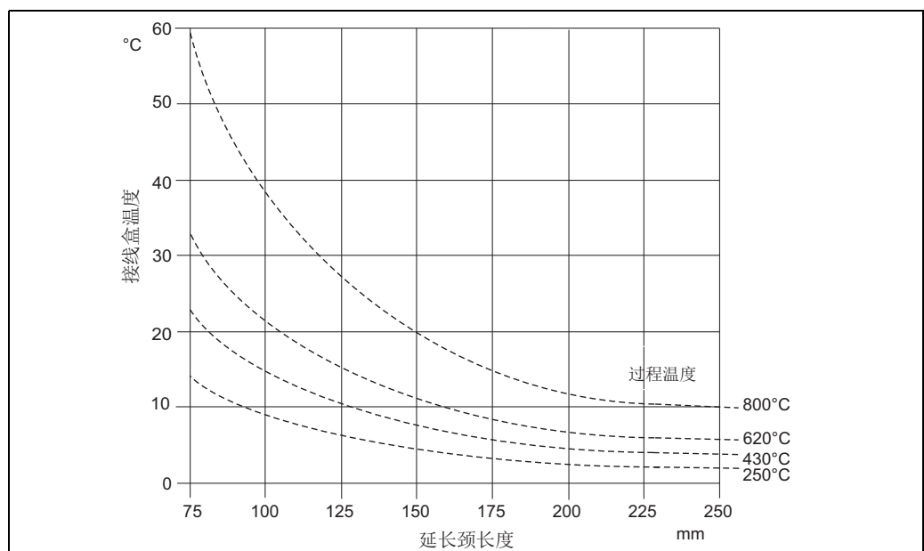
图 5: 接线盒温度 - 过程温度的关系曲线图
