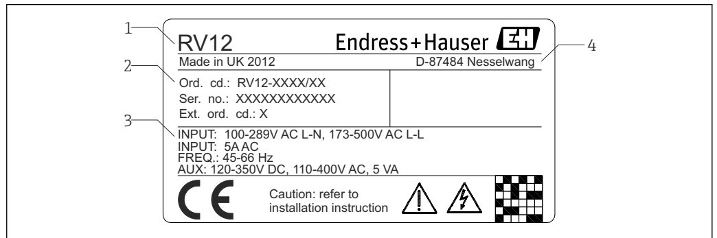
1 Typenschild EngyVolt RV12 (beispielhaft)
