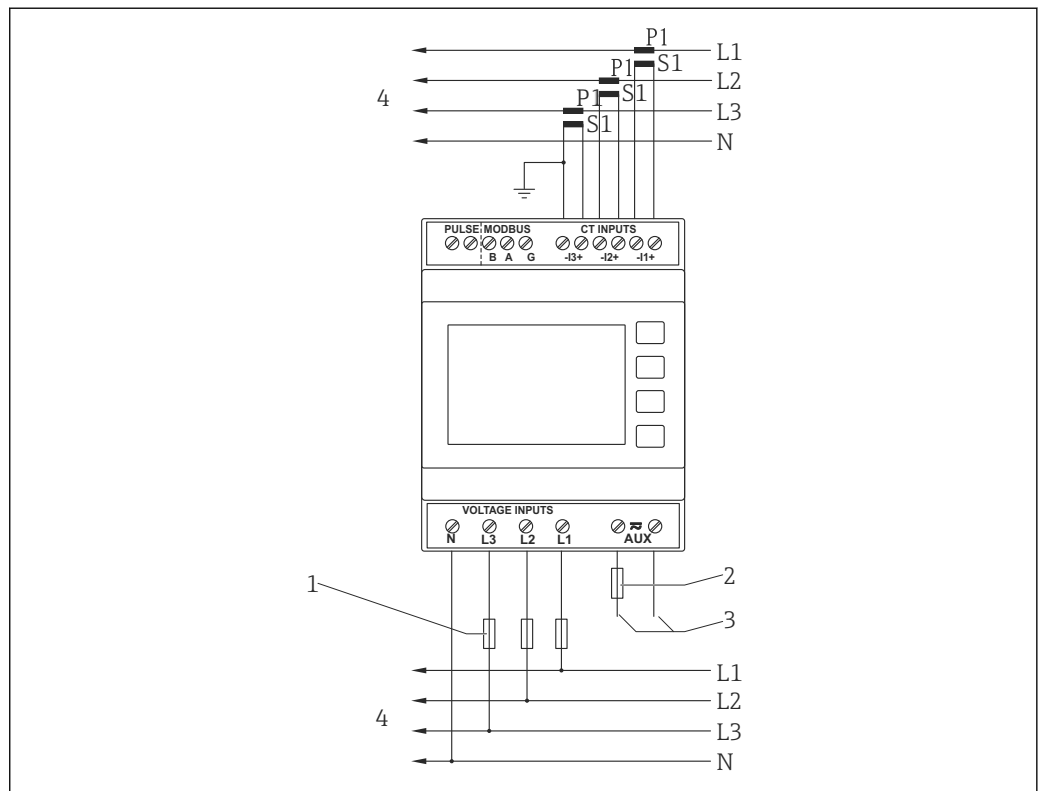
5 Anschluss im 3 Phasen 4 Leiter Netz
