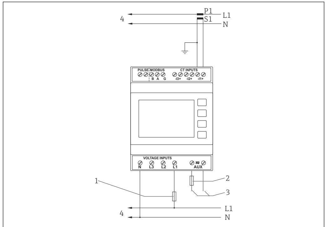
3 Anschluss im 1 Phase 2 Leiter Netz
