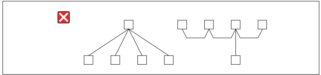
10 Falsche Stern- oder Abzweigverdrahtung
