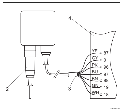
VS 接线盒与盘装型设备的连接示意图
