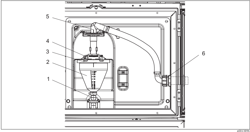
Abb. 1: Membranpumpe
