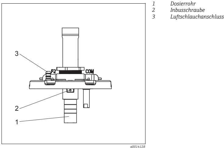
Abb. 2: Membranpumpe
