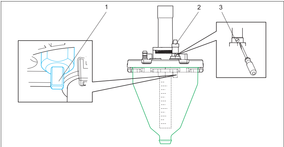
Abb. 3: Kapazitiven Sensor justieren
