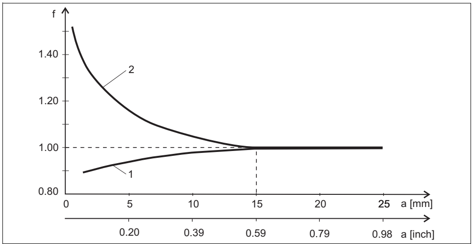
Abb. 7: Abhängigkeit des Einbaufaktors f vom Wandabstand
