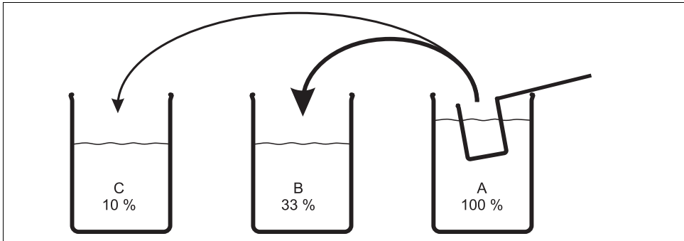
Abb. 8: Proben für eine Dreipunktkalibrierung herstellen
