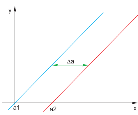
Abb. 6: Delta Nullpunkt bzw. Arbeitspunkt (ISFET-Sensor)
