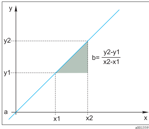
Abb. 4: Lineare Funktion
