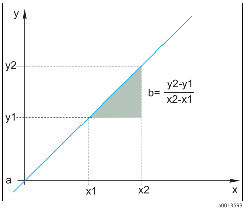
Fig. 4: Linear function
