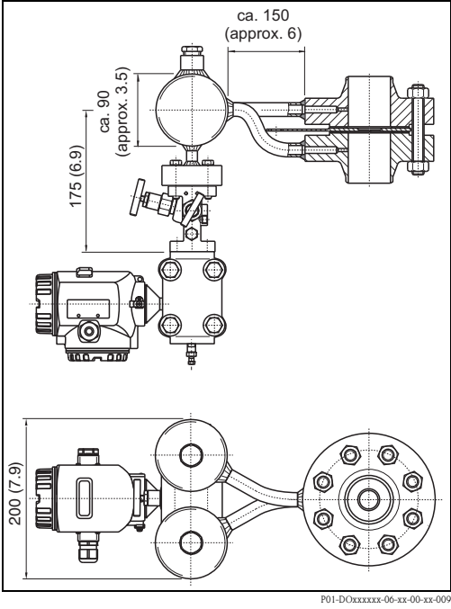
竖直管道中的蒸气测量； 尺寸：mm (inch)
