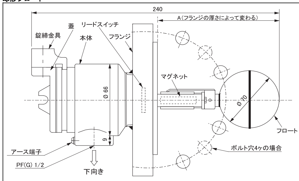
図 5: 球形フロートの寸法
