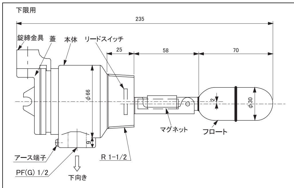
図 2: CS1103 の寸法
