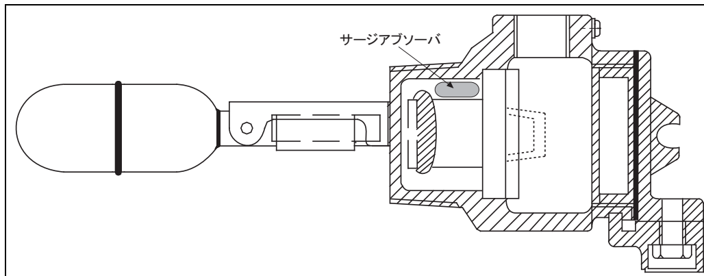
図 10: サージアブソーバ
