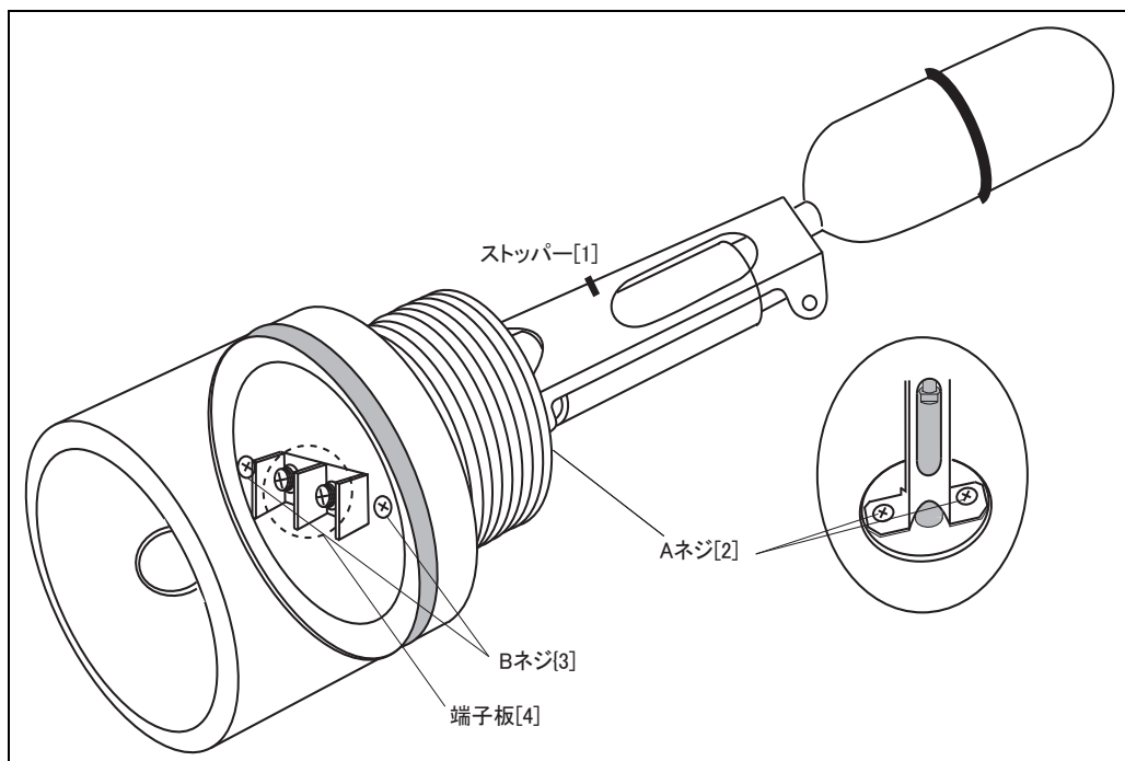
図 6: フロートスイッチ
