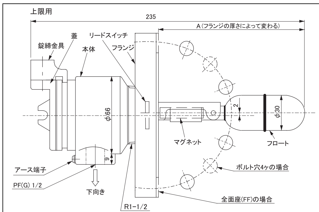
図 3: CS1203 の寸法
