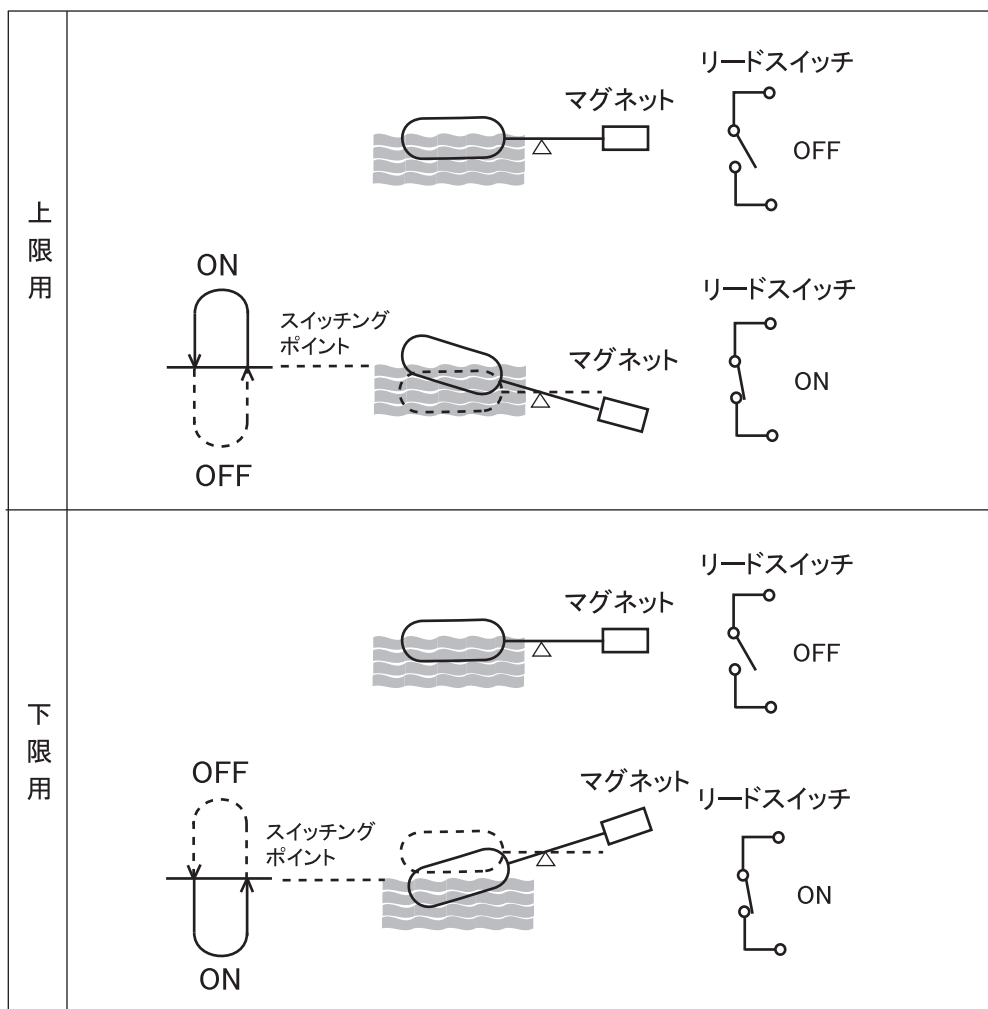
図 12: フロートレベルスイッチの動作
