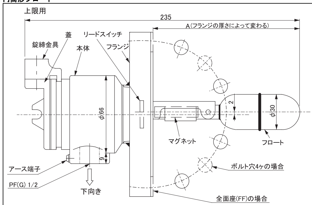
図 4: 円筒形フロートの寸法
