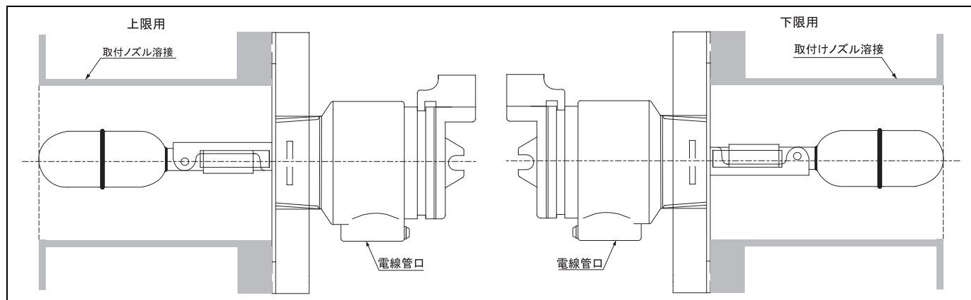
図 8: 円筒形フロートの取付け
