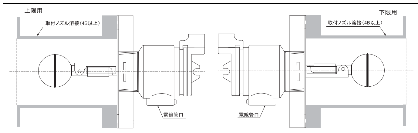
図 9: 球形フロートの取付け
