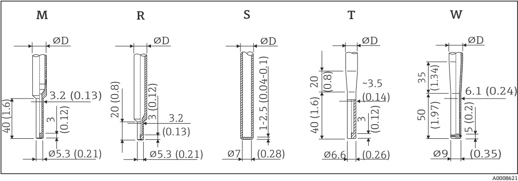
5 热保护套管末端类型(缩径型、直管型、锥管型)。最大表面光洁度 Ra \leq 0.8 \mu m (31.5 \mu in )
