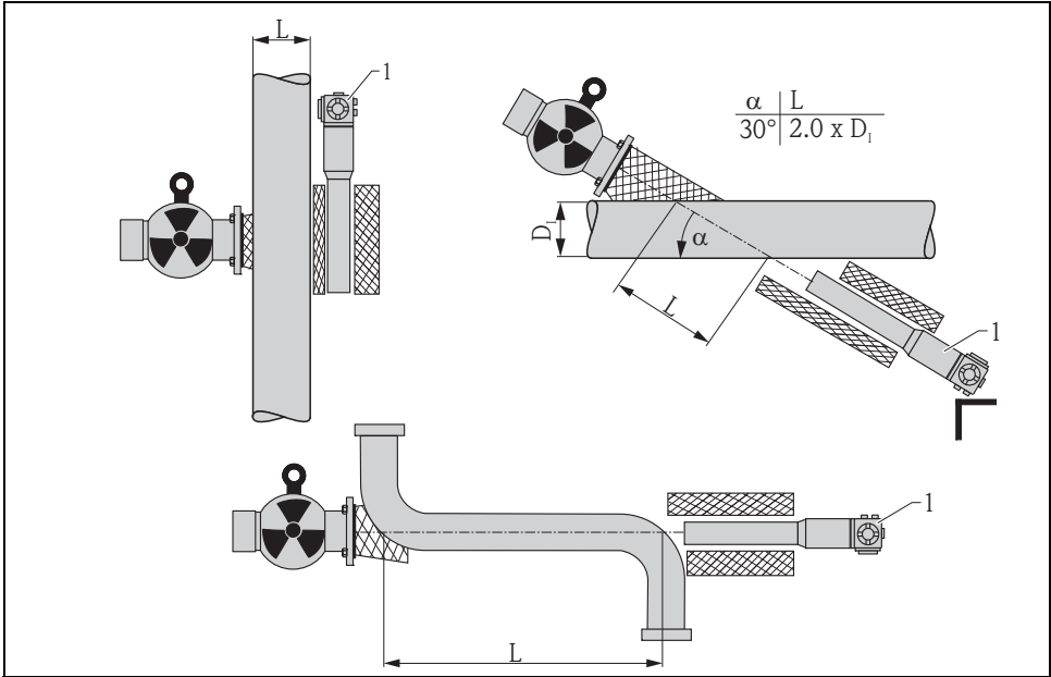
Toujours indiquer le chemin traversé L dans la fonction "Diamètre tube" (*0A). Selon l'installation, cette valeur peut être plus élevée que le diamètre effectif du tube.
