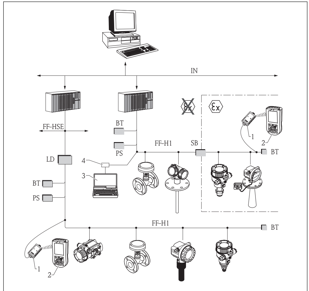
2 Architecture du système FOUNDATION Fieldbus avec composants associés
