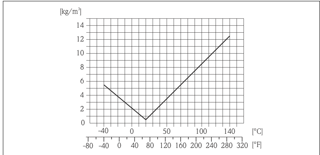
图 35 现场密度标定，例如：在+20 °C (+68 °F)时
