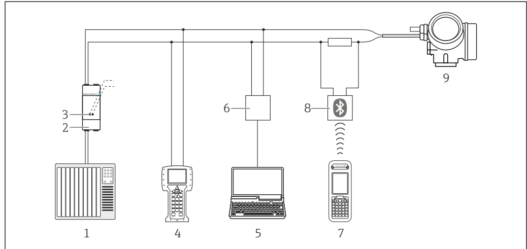
图 39 通过 HART 通信进行远程操作
