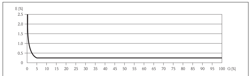
图 36 最大测量误差(% o.r.) (例如: DN 25)
