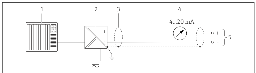
图 7 4...20 mA HART 无源电流输出的连接示例
