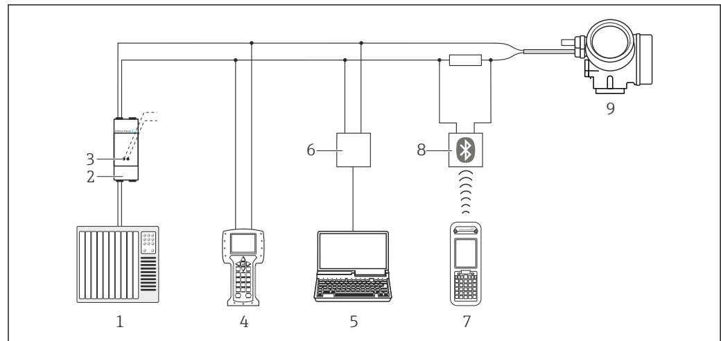
图 13 通过 HART 通信进行远程操作
