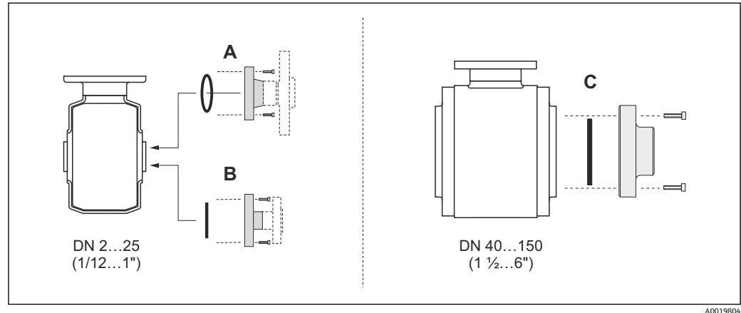
图 6 过程连接密封圈
