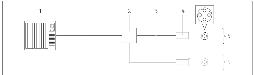
图 11 PROFINET 的连接电缆
