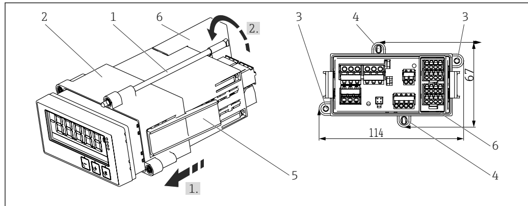
2 Einbau in Schalttafel
