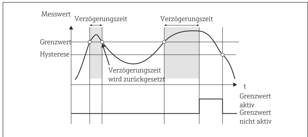
11 Hysterese und Verzögerung aktiv
