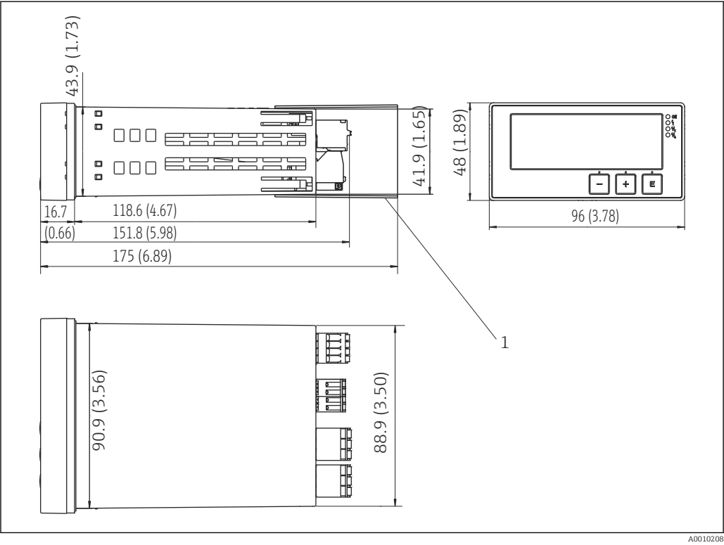
15 Abmessungen des Prozessanzeigers in mm (in)
