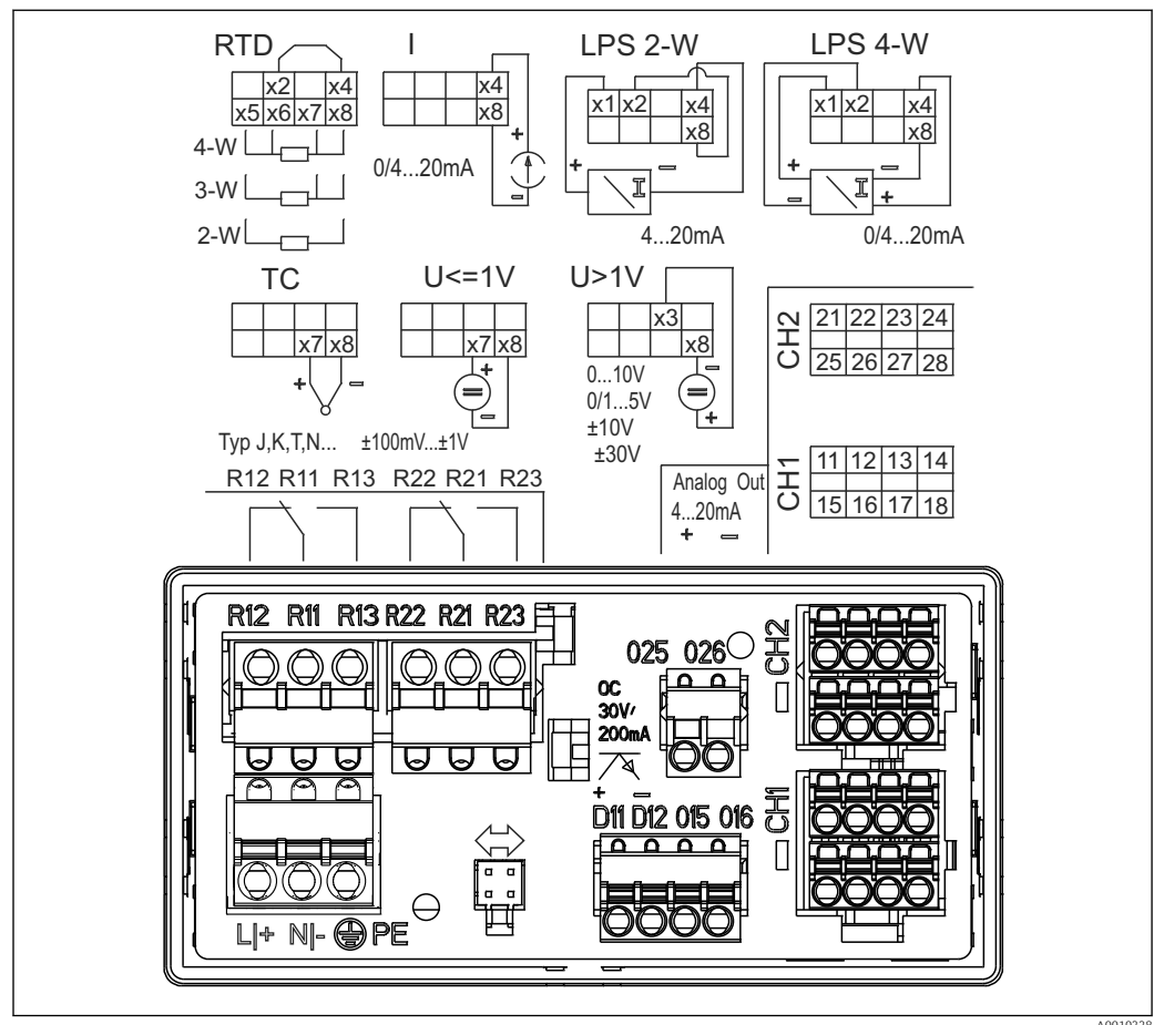
14 Klemmenbelegung des Prozessanzeigers (Relais (Klemmen Rx1-Rx3) und Kanal 2 (Klemmen 21-28 und 025/026) optional)
