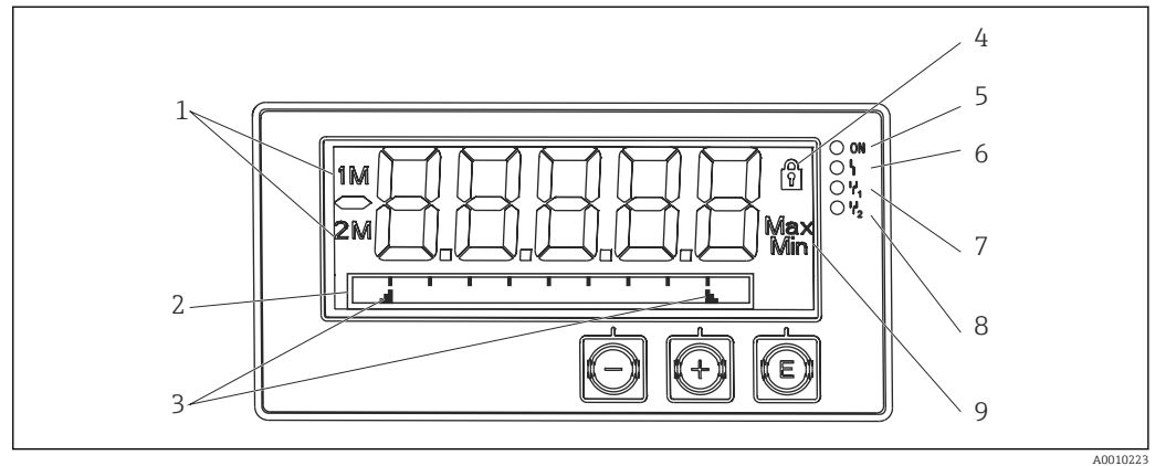
■ 16 Display des Prozessanzeigers
