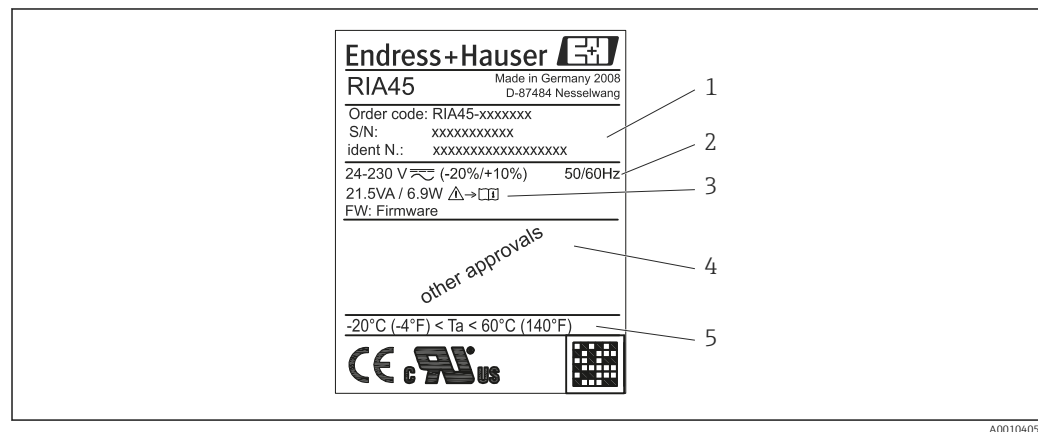
1 Typenschild des Prozessanzeigers (beispielhaft)
