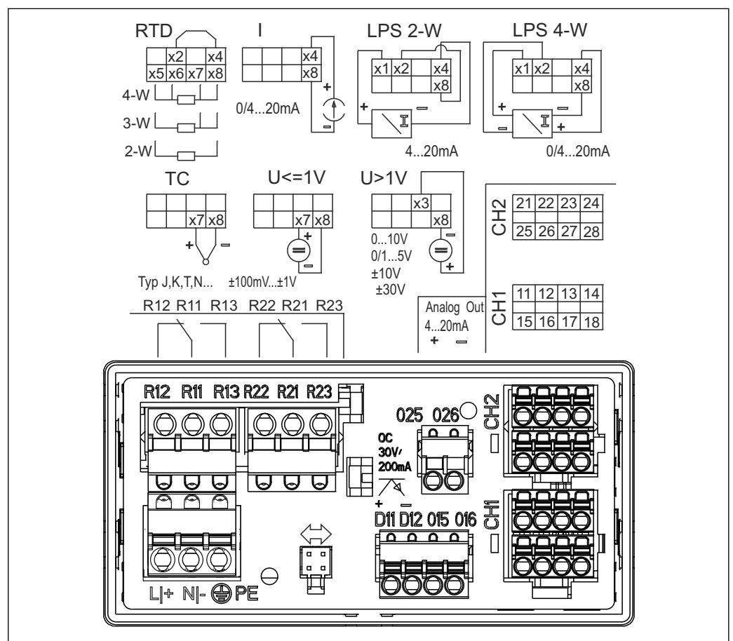
3 Anschlussbelegung des Geräts (Kanal 2 und Relais optional)
