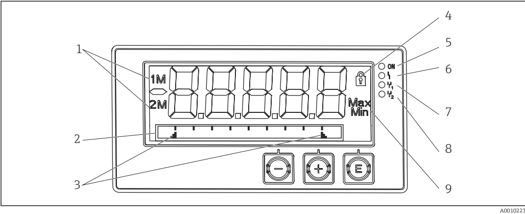
4 Display des Prozessanzeigers
