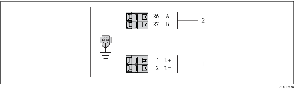
图 7 Modbus RS485 型仪表的接线端子分配示意图, 连接类型适用于在非危险区和 2 区/Div. 2 防爆场合中使用
