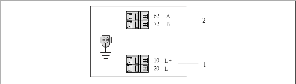
8 Modbus RS485 型仪表的接线端子分配示意图，连接类型适用于在本安防爆场合中使用(通过 Promass 100 安全栅连接)
