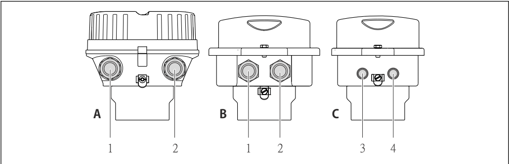
图 10 仪表类型和连接类型
