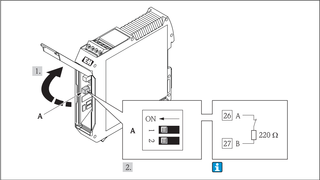
图 14 通过 Promass 100 安全栅上的 DIP 开关开启终端电阻
