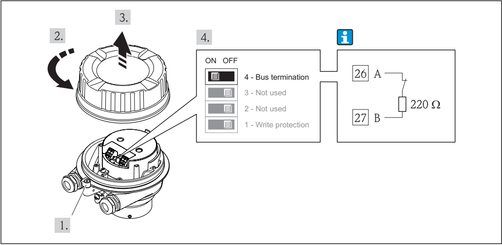
图 13 通过主要电子模块上的 DIP 开关开启终端电阻
