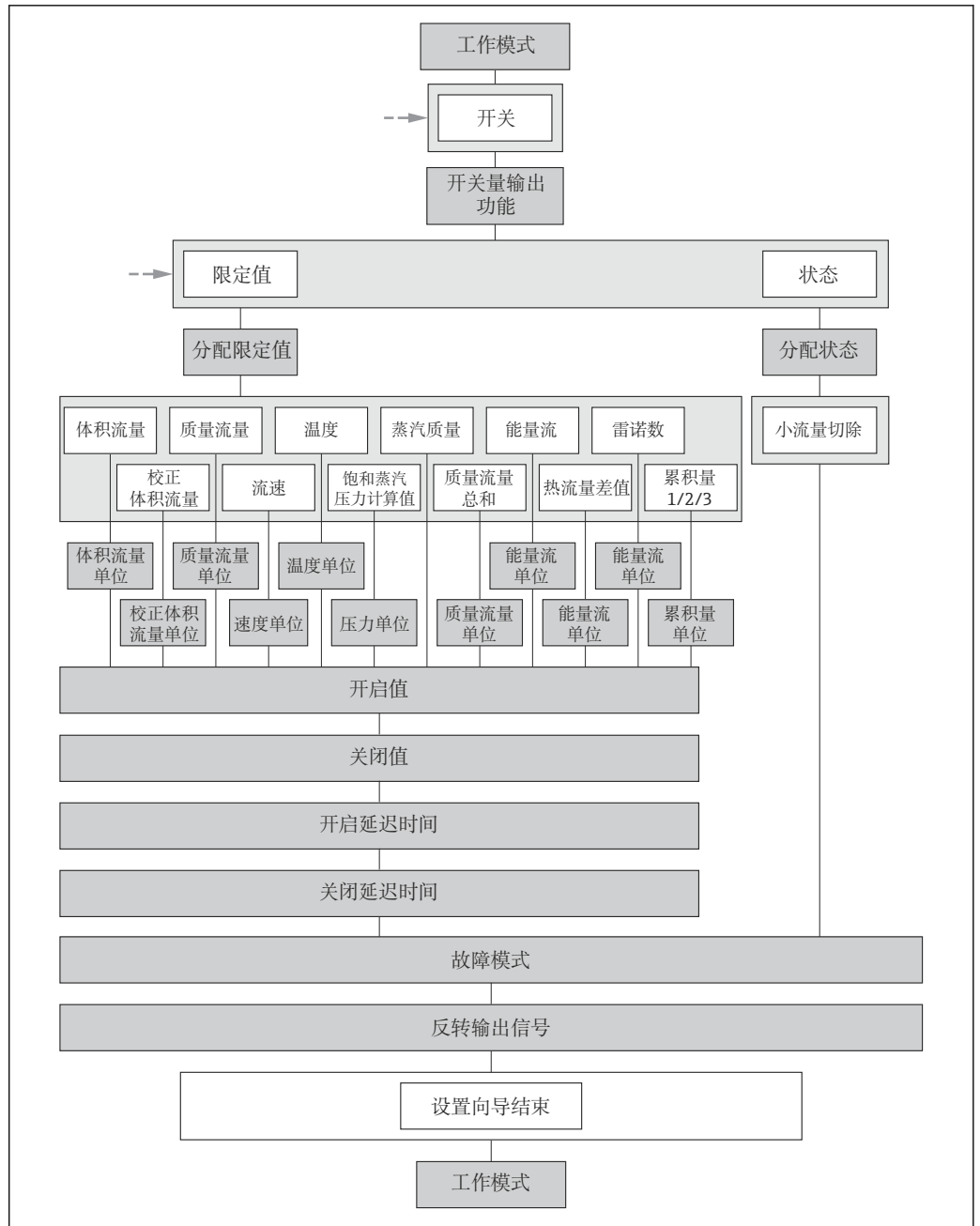
图 29 “脉冲/频率/开关 输出”向导(在“高级设置”子菜单中:“工作模式”参数“开关”选项) (第二部分)
