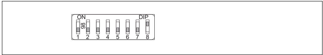
图 15 软件地址设定实例。开关 8 拨至“ON (开)”位置上；在操作菜单中设置地址(“设置”菜单→“通信”子菜单→“设备地址”参数)。
