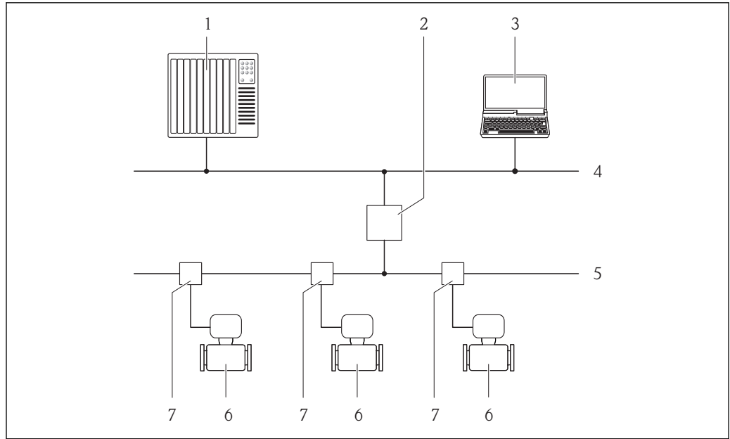
图 38 通过 PROFIBUS PA 网络进行远程操作
