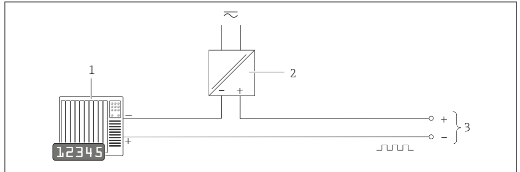
图 11 脉冲/频率输出(无源信号)的连接实例
