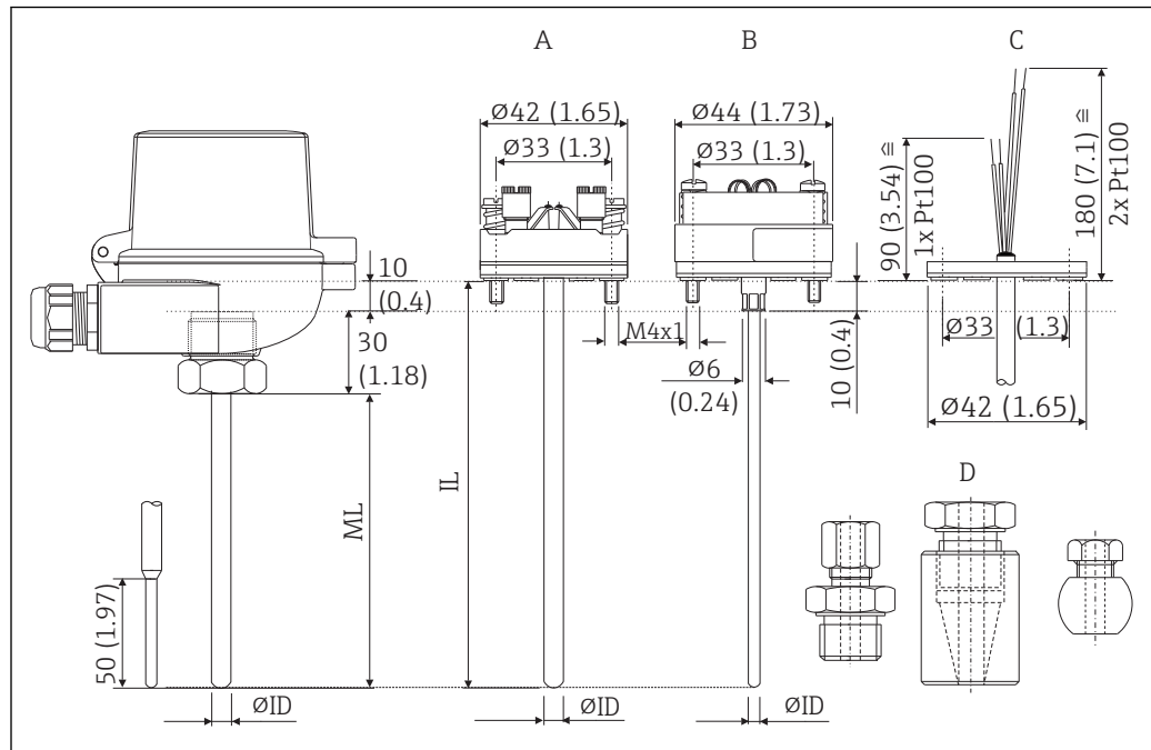
3 Abmessungen Omnigrad T TR24
