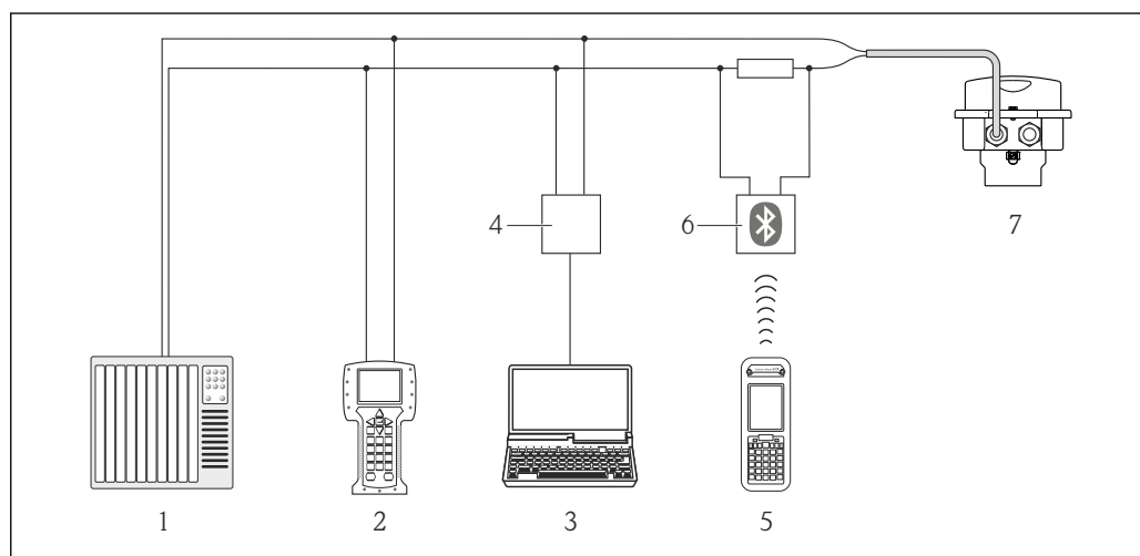
16 Possibilités de configuration à distance via protocole HART
