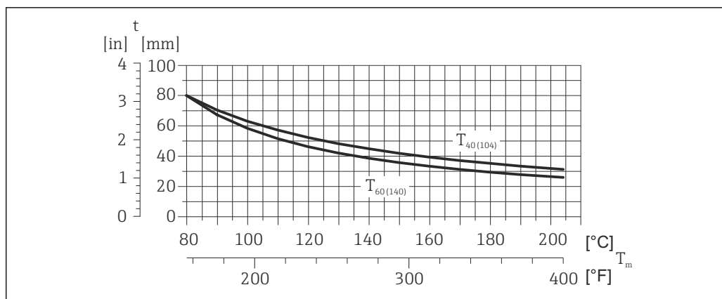
7 Epaisseurs d'isolation recommandées en fonction de la température du produit et ambiante
