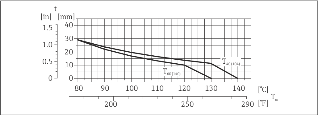
6 Epaisseurs d'isolation recommandées en fonction de la température du produit et ambiante
