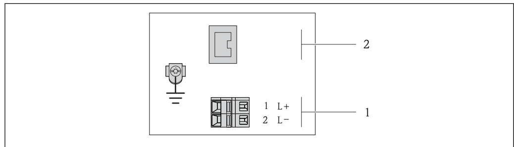
图 8 工业以太网(EtherNet/IP)的接线端子分配示意图
