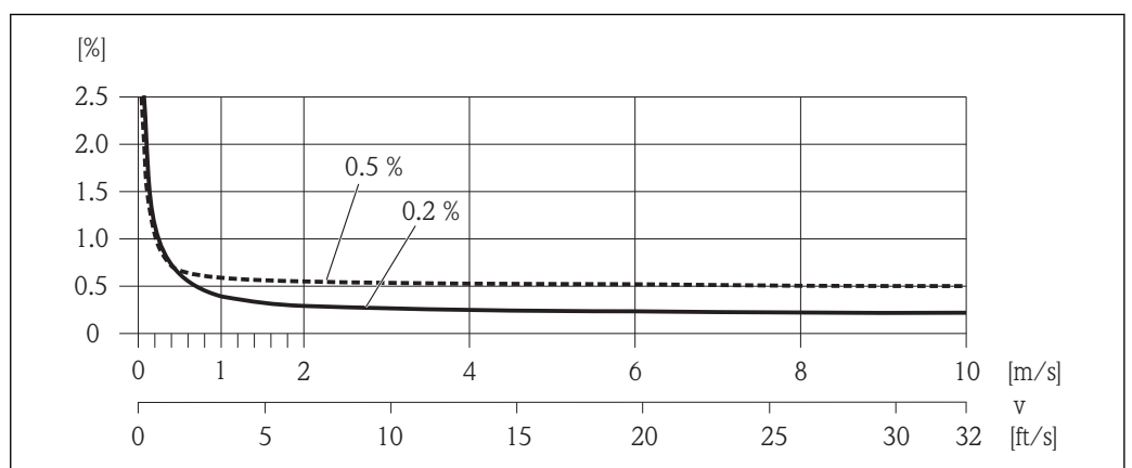
图 15 最大测量误差(% o.r.)示意图
