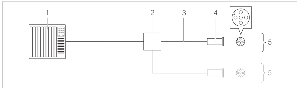
图 11 工业以太网(EtherNet/IP)的连接示例
