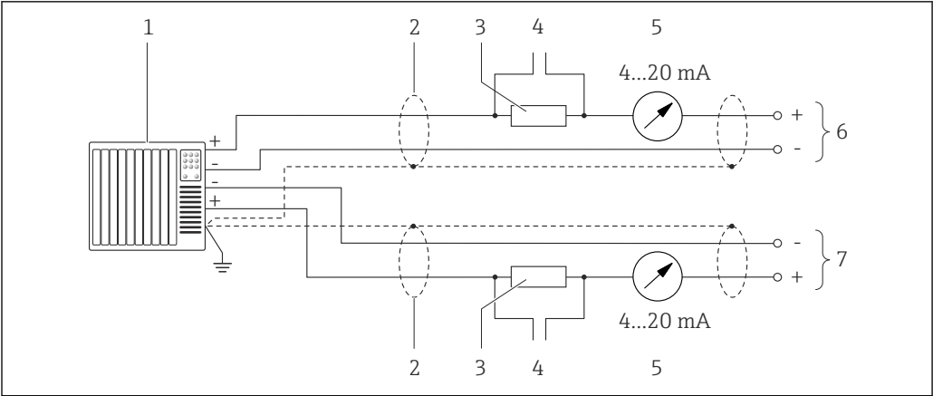
15 HART 输入(主站模式)的连接示例，通过有源电流输出
