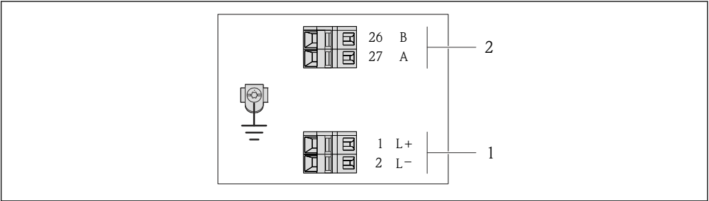
4 Modbus RS485 型仪表的接线端子分配示意图
