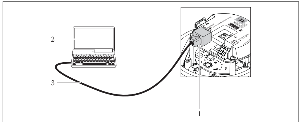
图 32 订购选项“输出”，选型代号 N: 工业以太网(EtherNet/IP)
