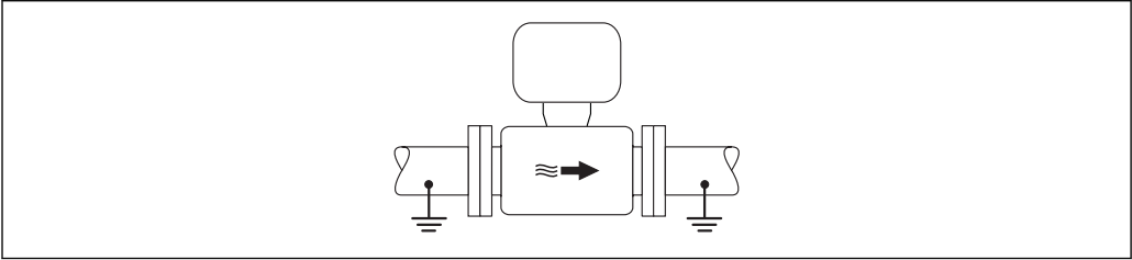
16 通过测量管实现电势平衡
