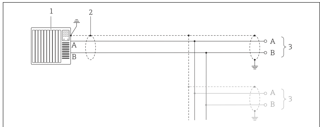
图 10 PROFIBUS DP 的连接示例，在非危险区和 2 区/ Div. 2 防爆场合中
