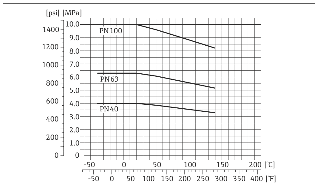
図 24 フランジ材質 1.4404 (SUS F316 または F316L 相当)
