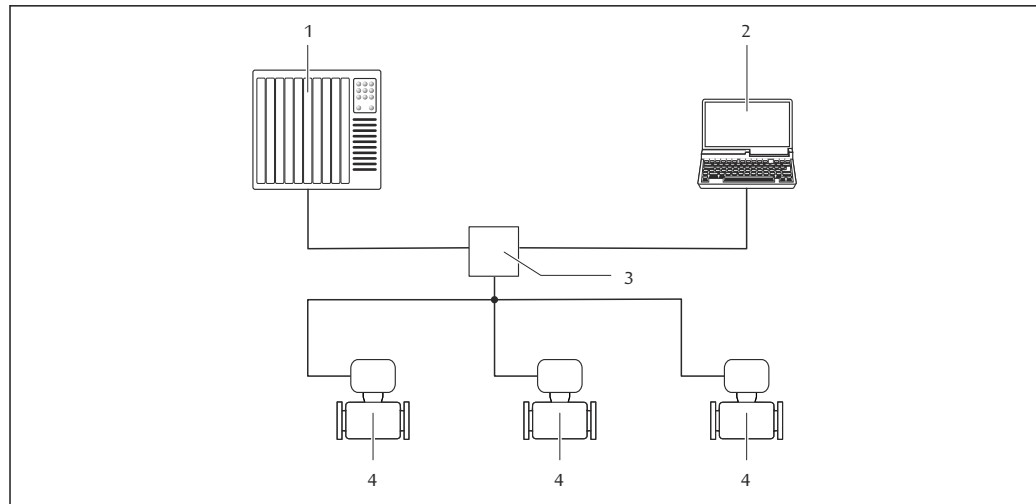
図 47 PROFINET ネットワーク経由のリモート操作オプション
