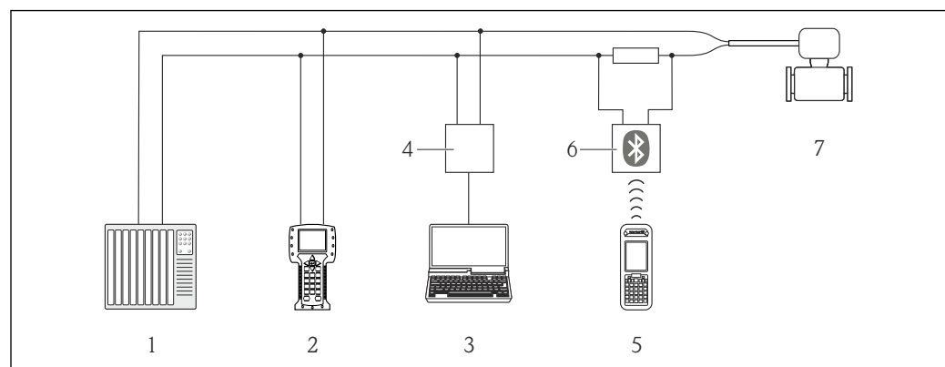
図 44 HART 経由のリモート操作オプション
