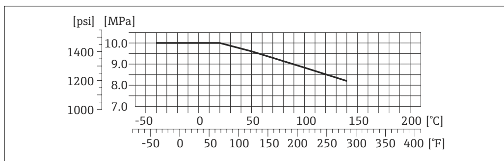
図 32 接続部の材質 1.4404 (SUS 316 または 316L 相当)
