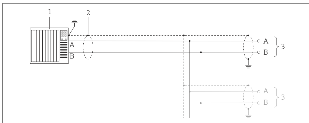
図 12 PROFIBUS DP（非危険場所および Zone 2/Div. 2 用）の接続例
