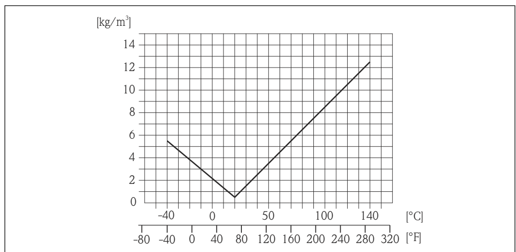
19 現場密度校正、+20 °C (+68 °F) 時の例
