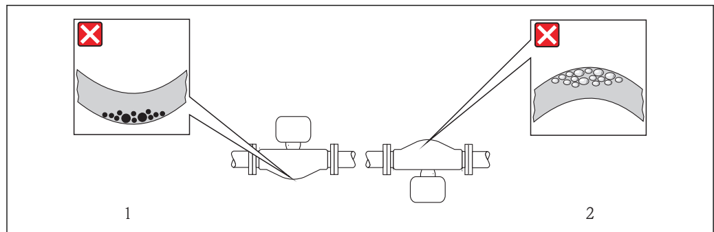
☒ 21 弓形計測チューブセンサの取付方向
