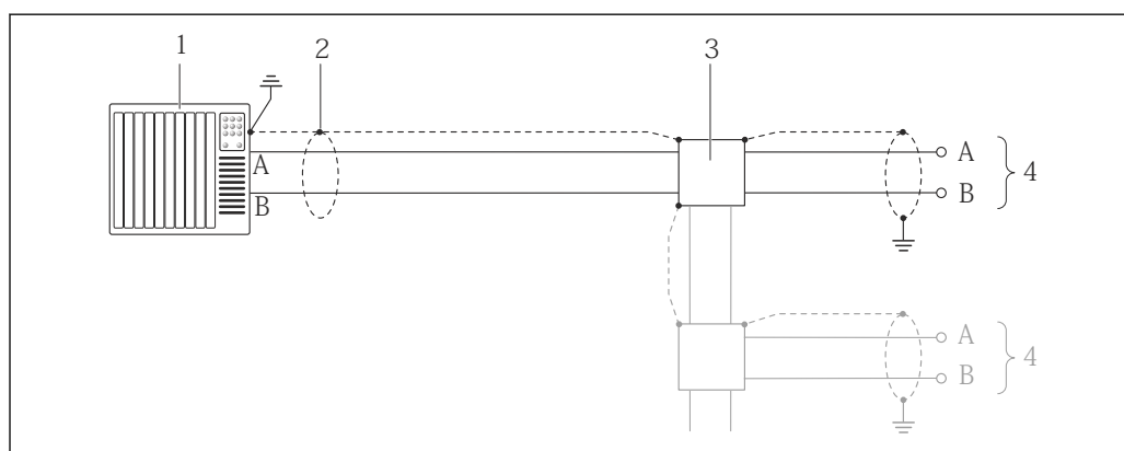
図 13 Modbus RS485（非危険場所および Zone 2/Div. 2 用）の接続例
