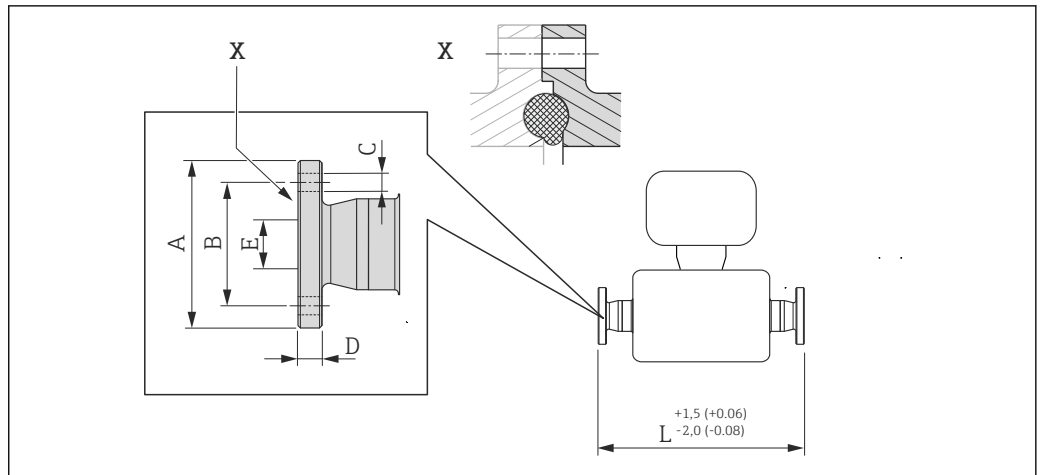
図 34 Xの詳細：非対称型プロセス接続；組み合わせクランプ、Oリングはお客様でご用意ください。 単位 mm (in)
