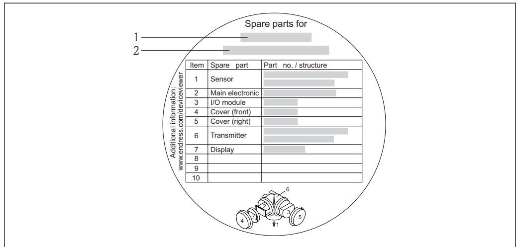
图 37 接线腔盖中的“备件概述图标”示例
