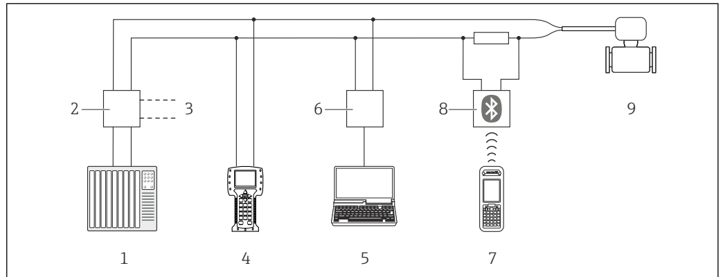
图 40 通过 HART 通信进行远程操作
