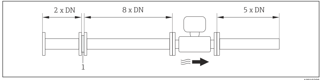
1 流量调节器
