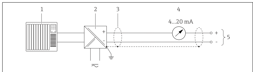
图 12 4...20 mA HART 无源电流输出的连接示例
