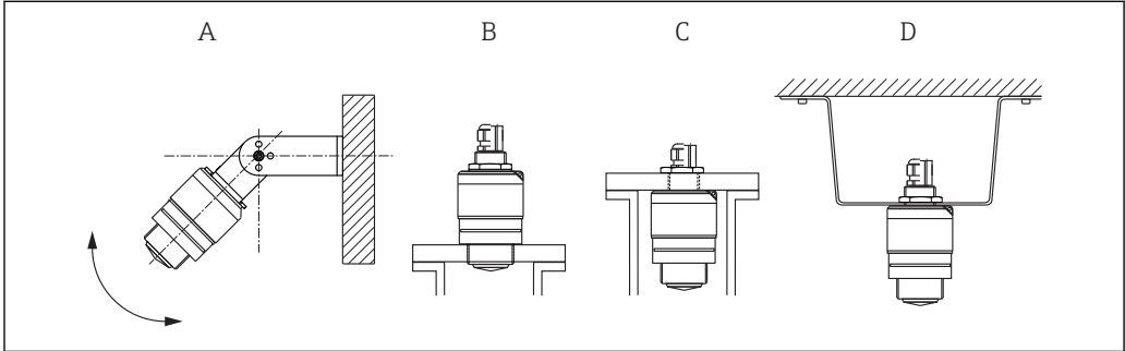
图 3 壁式安装、罐顶安装或安装短管安装 A 壁式安装或罐顶安装，可调节 B 螺纹安装(正面) C 螺纹安装(背面) D 使用对接螺母进行罐顶安装(对接螺母是标准供货件)
