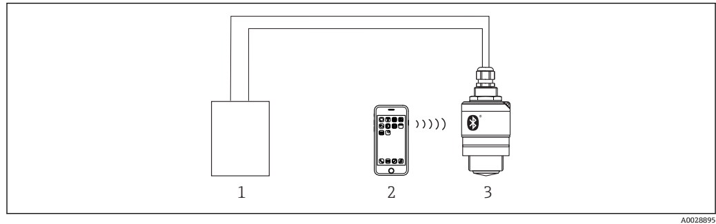
图 15 通过 Bluetooth®无线技术进行远程操作
