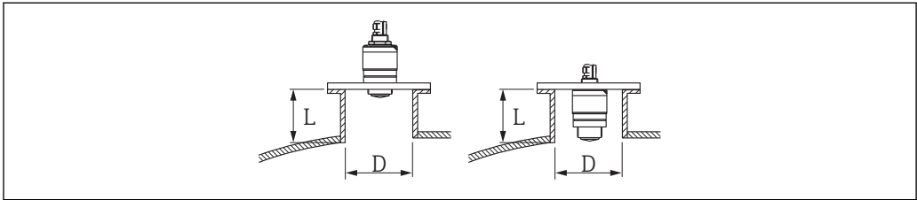
图 4 在安装短管中安装 FMR10
