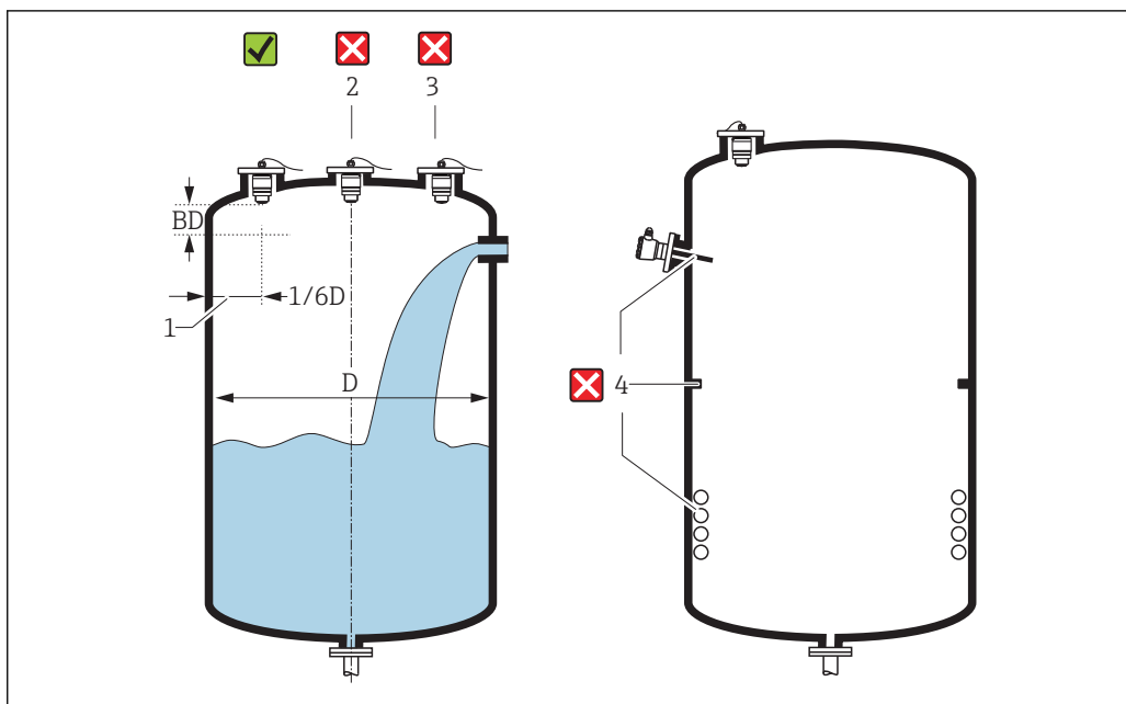
图 5 罐体上的安装位置
