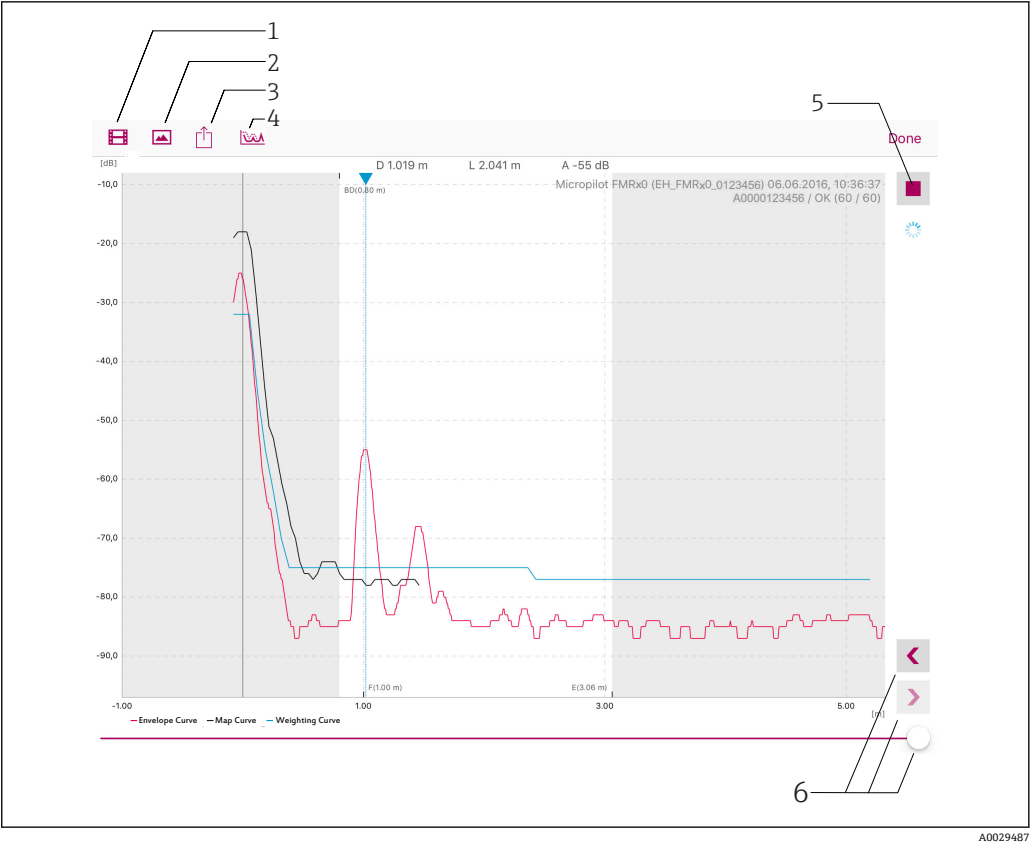
图 21 iOS 界面
